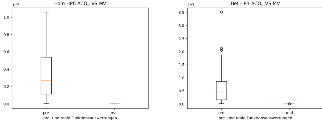
Abbildung 20: Verhältnis zwischen den benötigten Funktionsauswertungen für Vorfiltern, zusätzlichem Filtern und realen Iterationsschritten der Algorithmen für den Fall „exact-penalty“ und NSS-adapt, Teil 1
