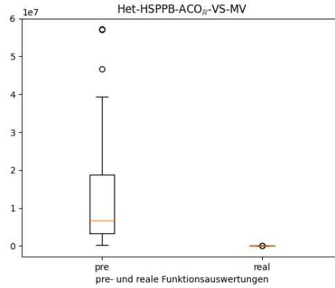
Abbildung 21: Verhältnis zwischen den benötigten Funktionsauswertungen für Vorfiltern, zusätzlichem Filtern und realen Iterationsschritten der Algorithmen für den Fall „exact-penalty“ und NSS-adapt, Teil 2
