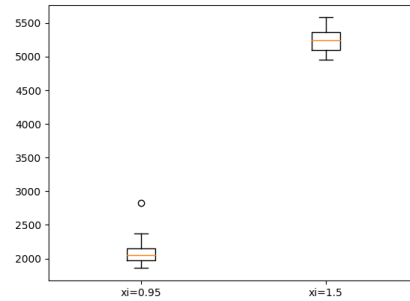
(b) \text{ACO}_{\mathbb{R}}\text{-very-simple}
