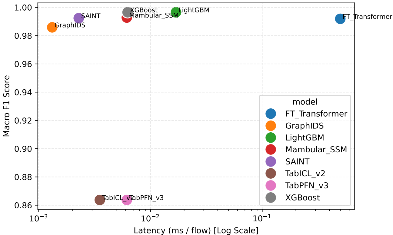
Pareto Frontier: CIC-DDOS2019 (Track A)
