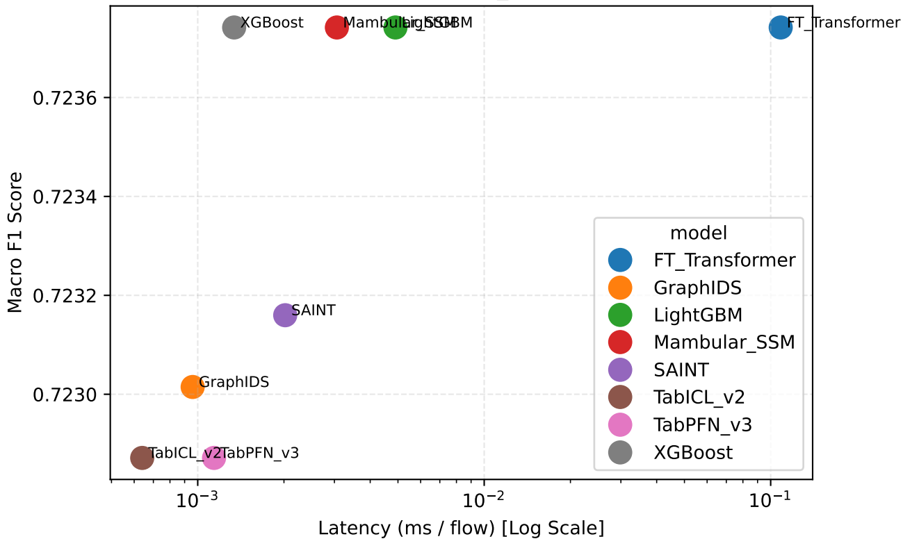
Pareto Frontier: TON_IOT (Track A)
