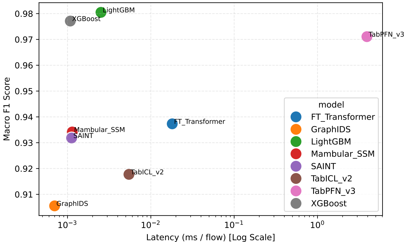
Pareto Frontier: CICIDS2017 (Track A)
