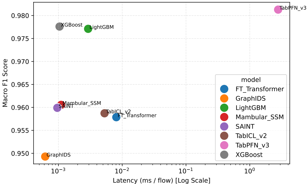
Pareto Frontier: NSL-KDD (Track A)
