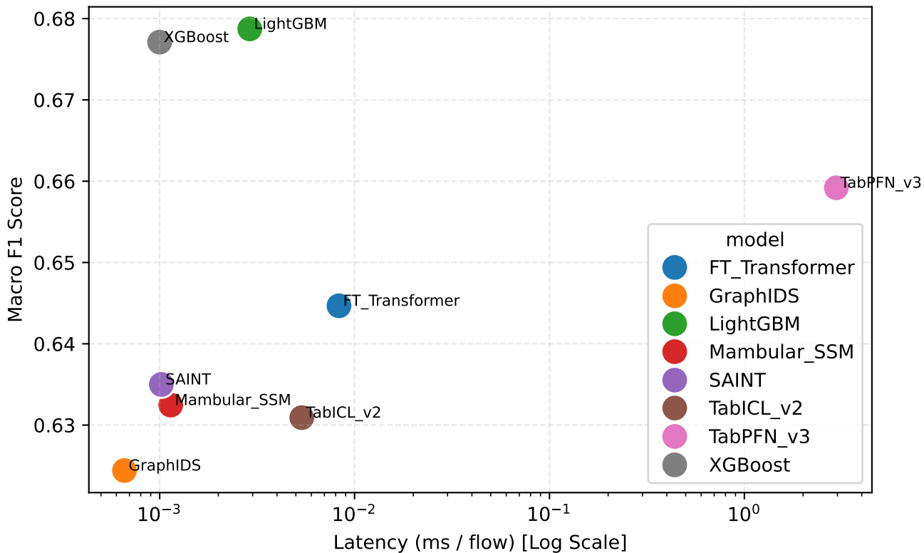
Pareto Frontier: UNSW-NB15 (Track A)
