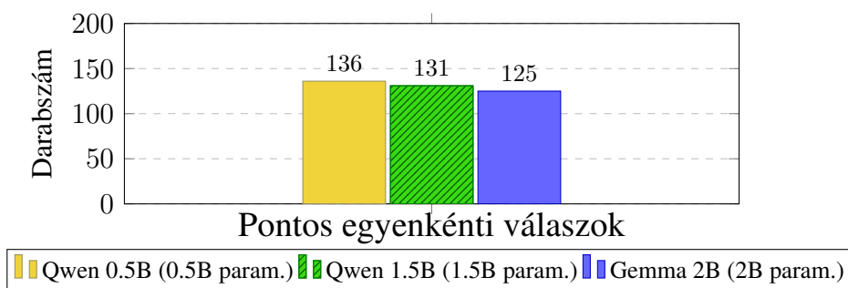
5.2. ábra. Három modell pontos egyenkénti válaszainak (gold standard címkékkel való egyezések) összehasonlítása ugyanezen a 200 véletlenszerű kérdé- désen.
