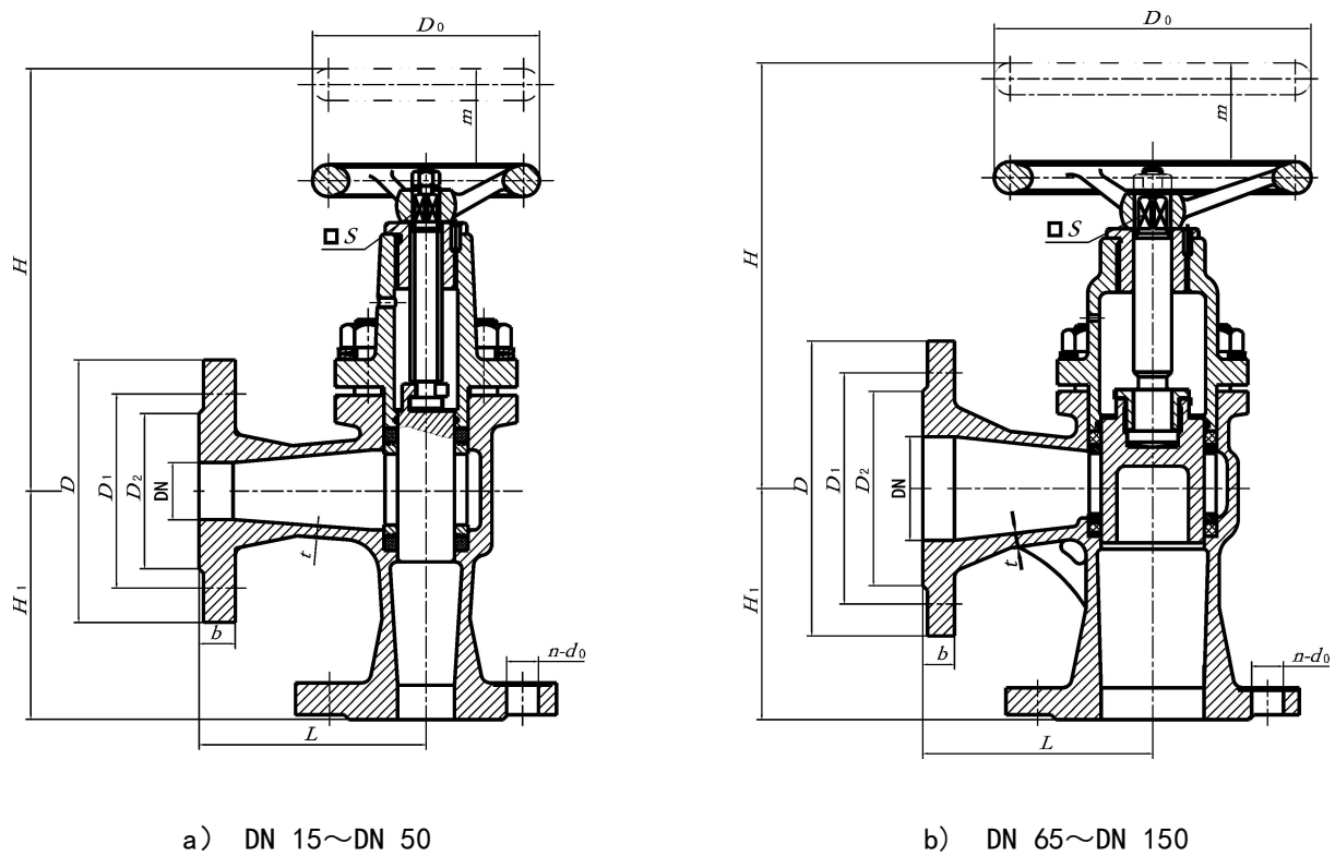
图 2 B 型、BS 型柱塞阀
