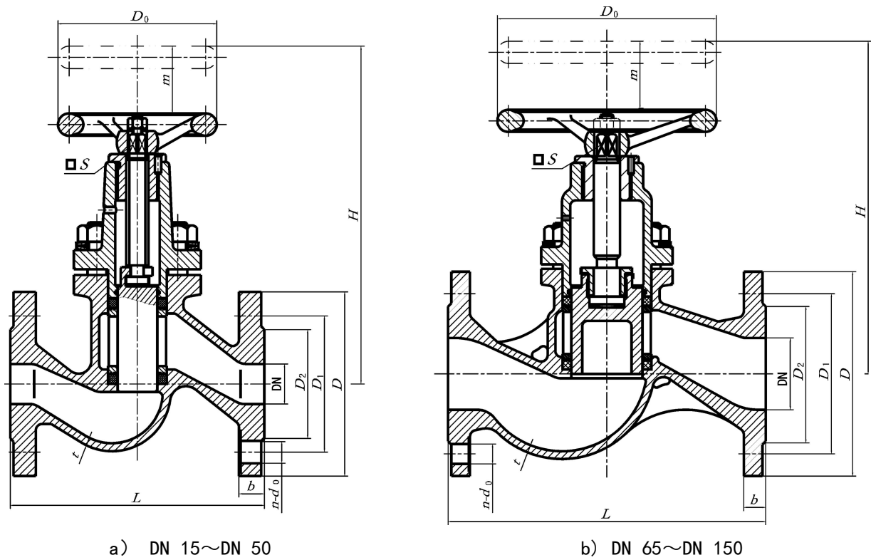
图 1 A 型、AS 型柱塞阀
