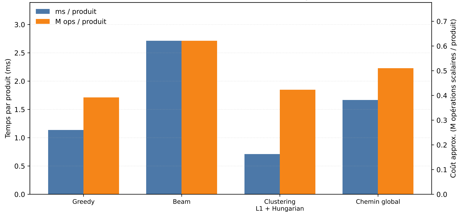
Coût d'inférence L2-L7 - Qwen3-Embedding-0.6B
