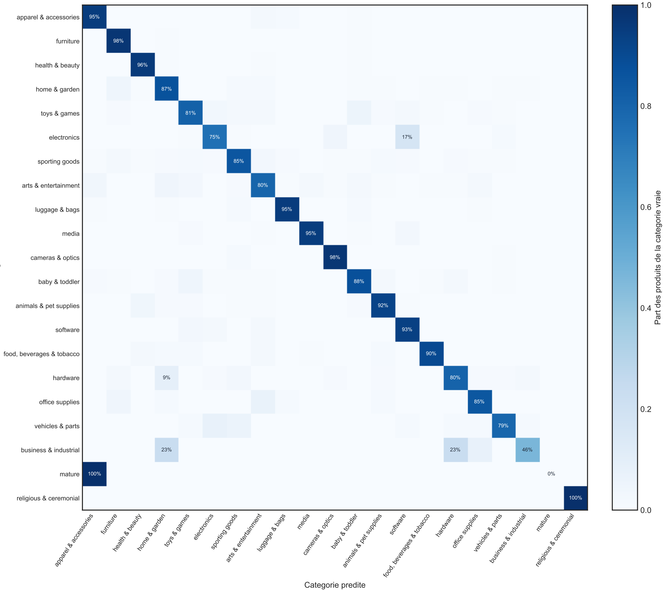
Matrice de confusion normalisee par categorie vraie
