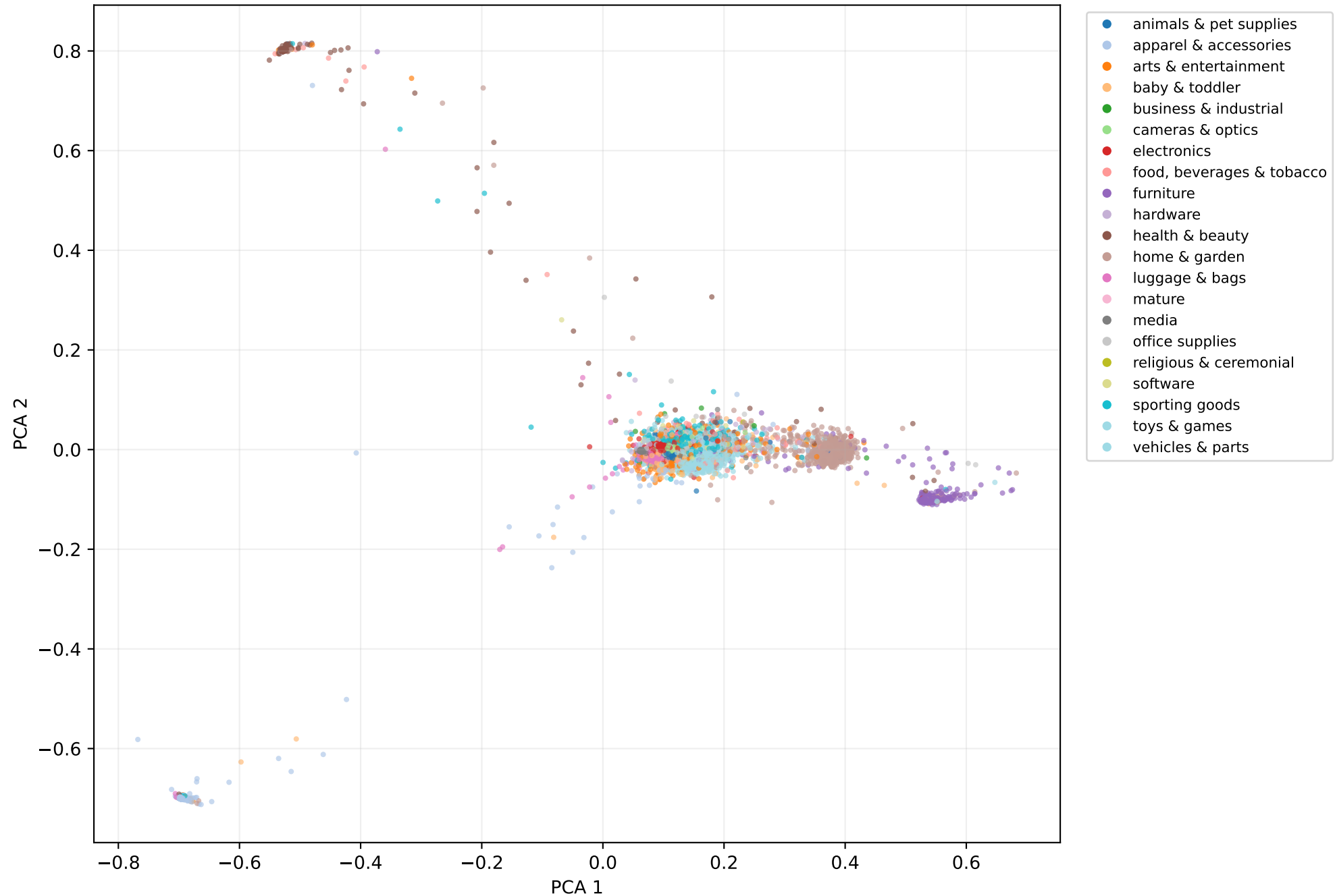
Projection 2D des embeddings produits L1 (PCA)
