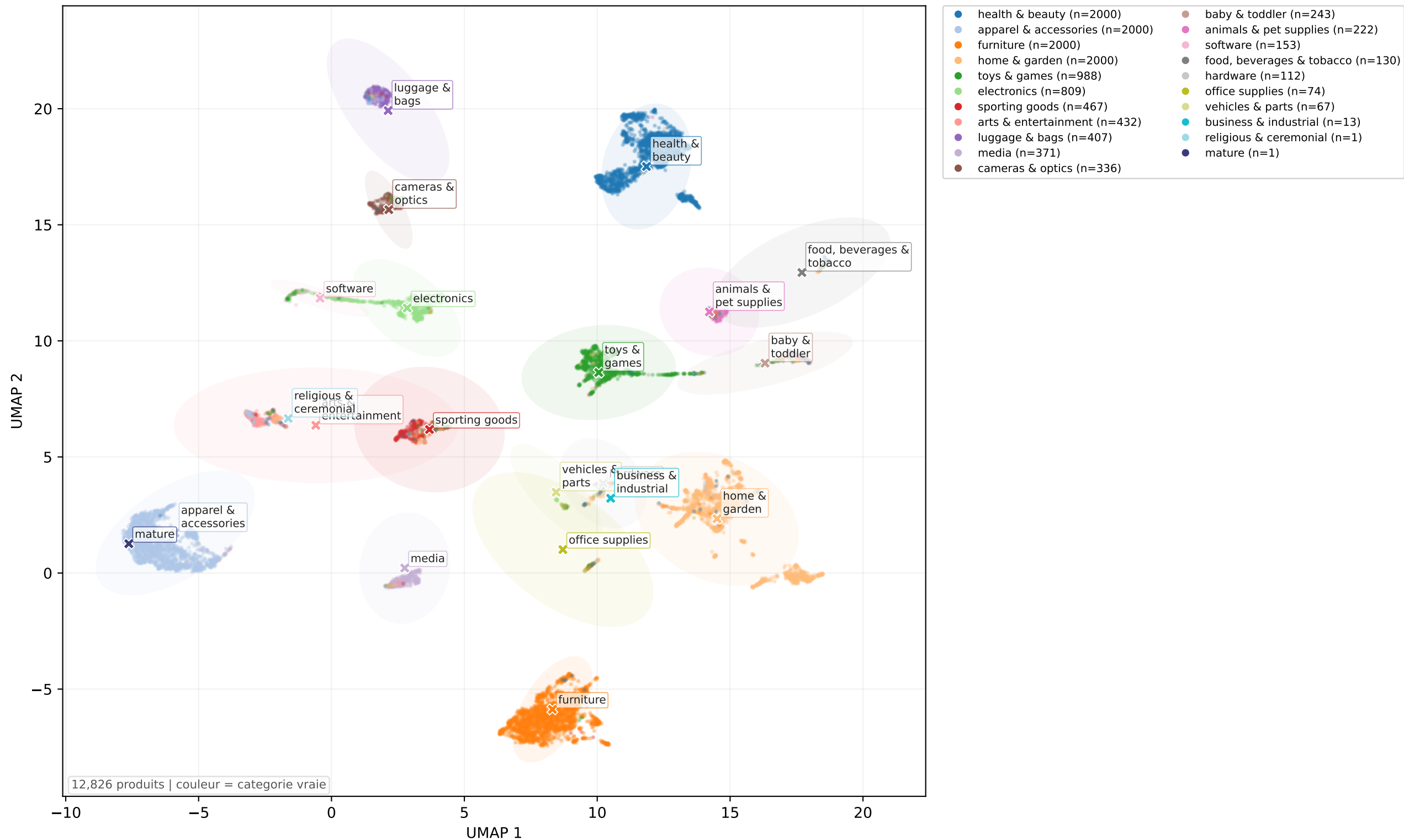
Projection 2D des embeddings produits L1 (UMAP)
