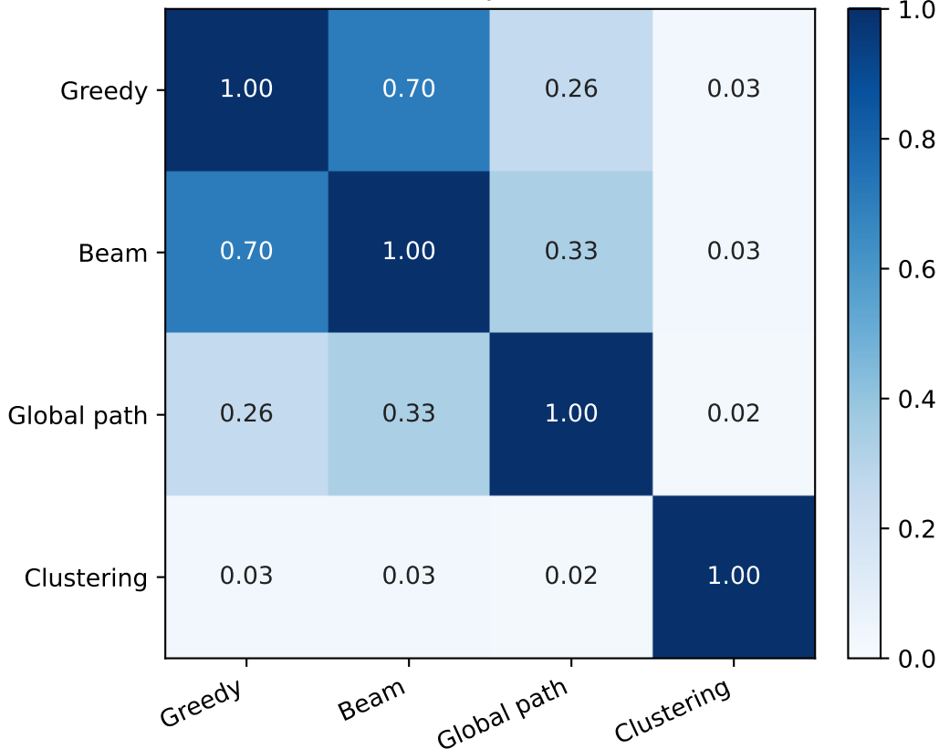
Accord exact sur le chemin complet - Qwen3, n=500 désaccords
