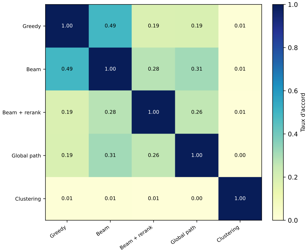
JASPER - accord exact au niveau L4
