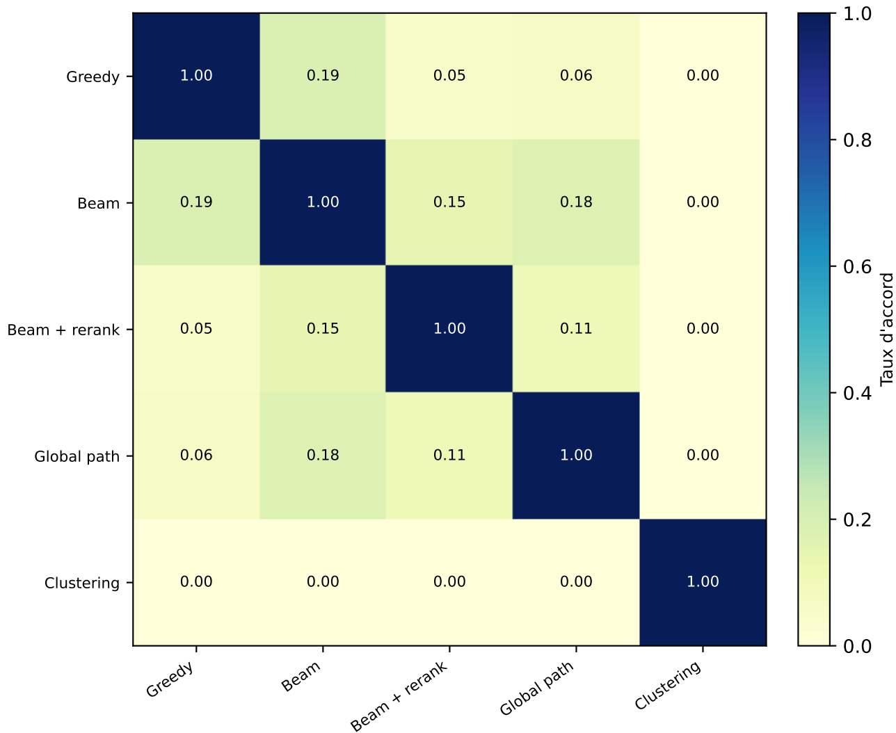
JASPER - accord exact au niveau L6
