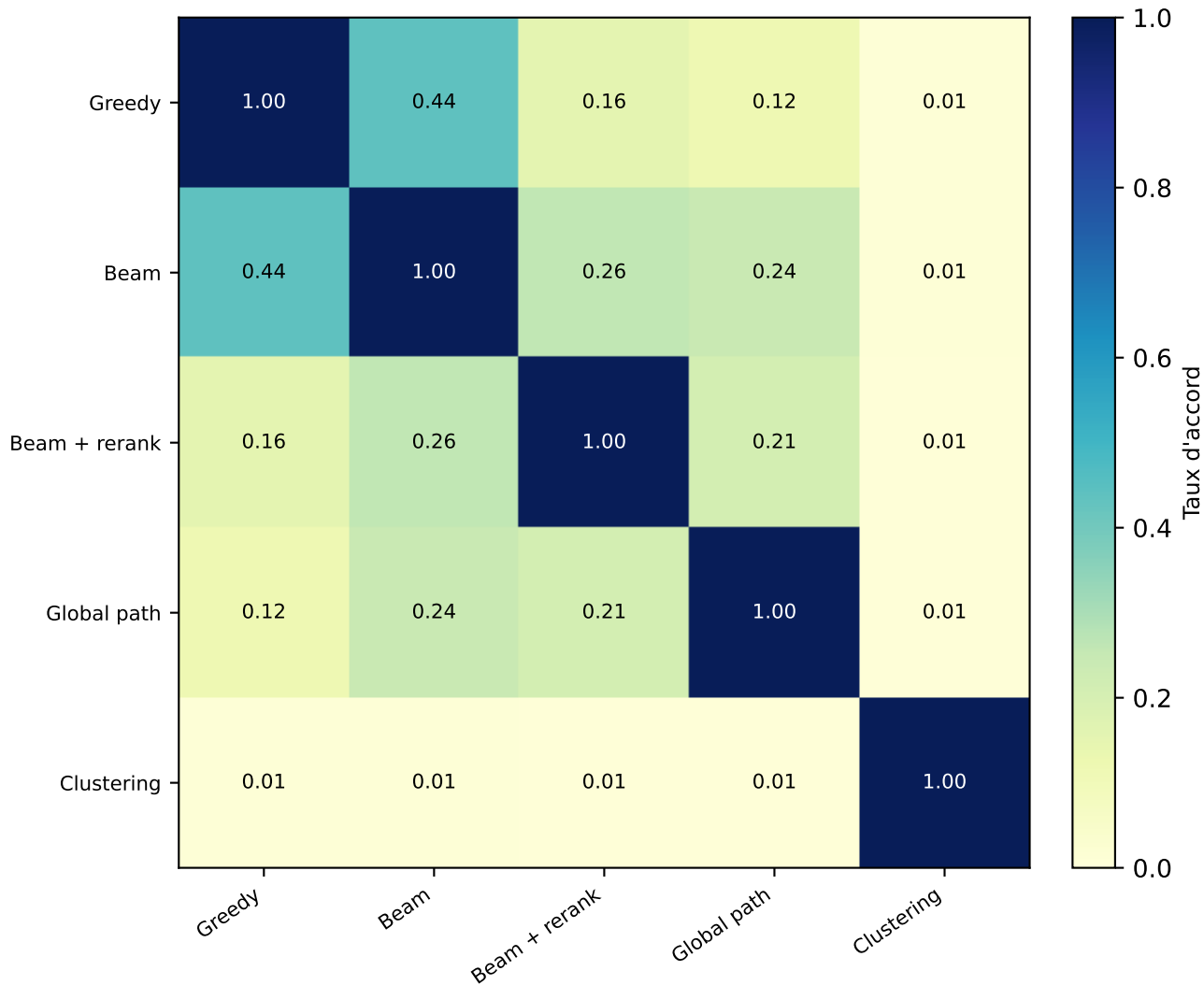
QWEN - accord exact au niveau L4
