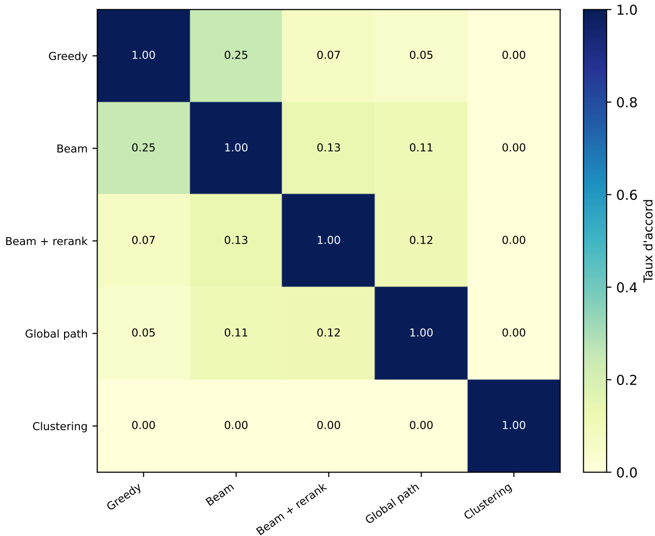
QWEN - accord exact au niveau L6
