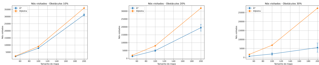
Figura 1. Nós visitados em função do tamanho do mapa para densidades de 10%, 20% e 30% de obstáculos (média ± desvio padrão sobre 30 sementes).
