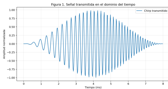
(a) Señal transmitida.
