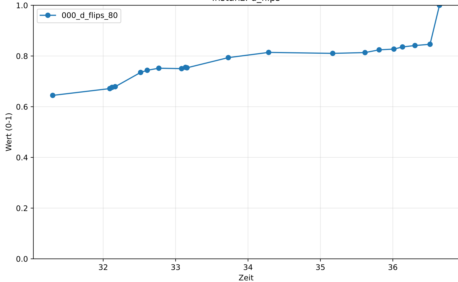
Instanz: d_flips
