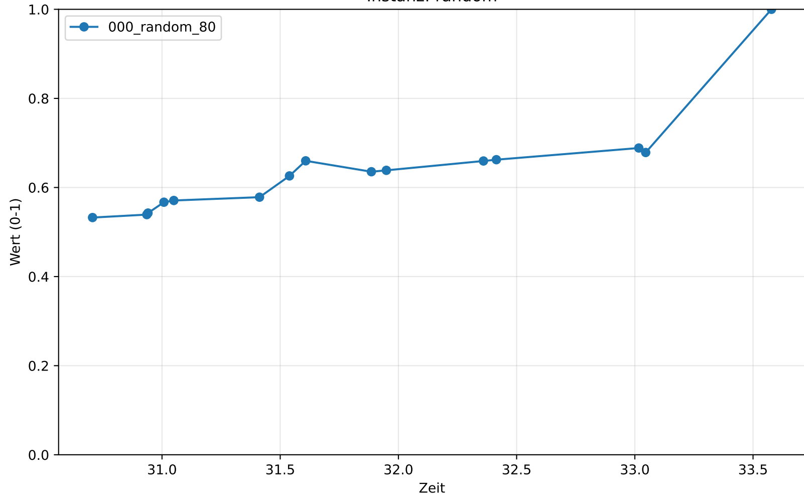
Instanz: random
