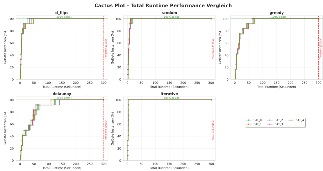
Abbildung A.3.: Es ist zu sehen das SAT bei mehreren Permuation vor allem bei den delaunay leicht unterschiedliche Laufzeiten hat.
