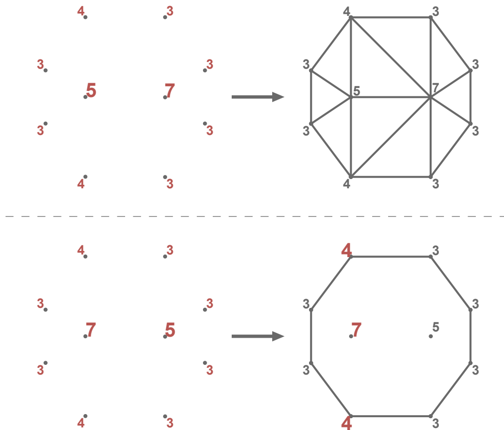
Abbildung 1.1.: Eine Ja-Instanz (oben) und eine Nein-Instanz (unten). Die Zahlen an den Knoten sind die Sollgrade. Bei der Nein-Instanz können die Sollgrade mit einer Triangulierung nicht eingehalten werden.
