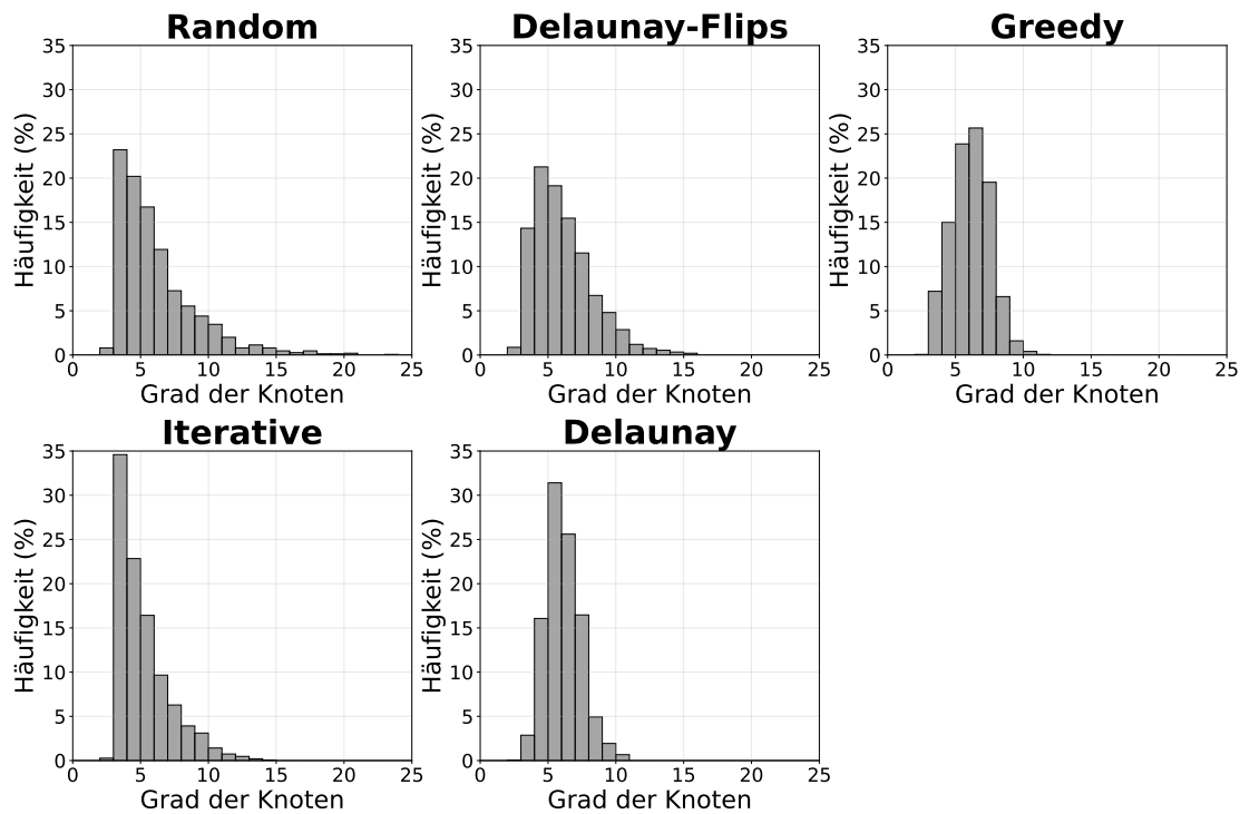
Abbildung 4.10.: In dieser Abbildung ist die Gradverteilung der Knoten pro Instanz zu sehen.
