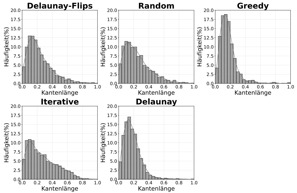
Abbildung 4.11.: In dieser Abbildung ist die Verteilung der Kantenlängen pro Instanz zu sehen. Dabei sind die Kantenlängen normiert, sodass sie zwischen 0 und 1 liegen. Dafür wurde alle Kantenlängen durch die maximale Kantenlänge geteilt.
