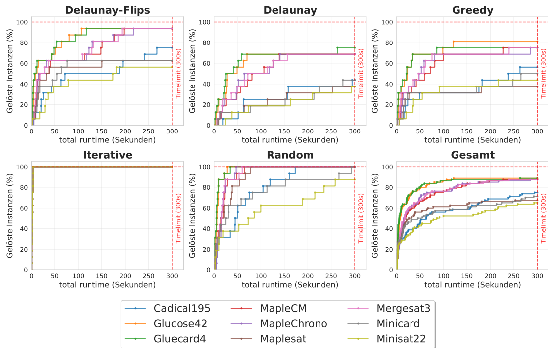
Abbildung 4.2.: In dieser Abbildung sind die Laufzeiten der verschiedenen SAT-Solver für die verschiedenen Instanzen zu sehen. Hierbei ist klar erkennbar dass Gluecard4 und Glucose42 die besten Ergebnisse erzielen.
