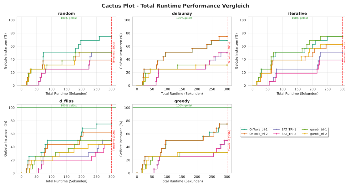
Abbildung 4.11: Eval Dreiecke
