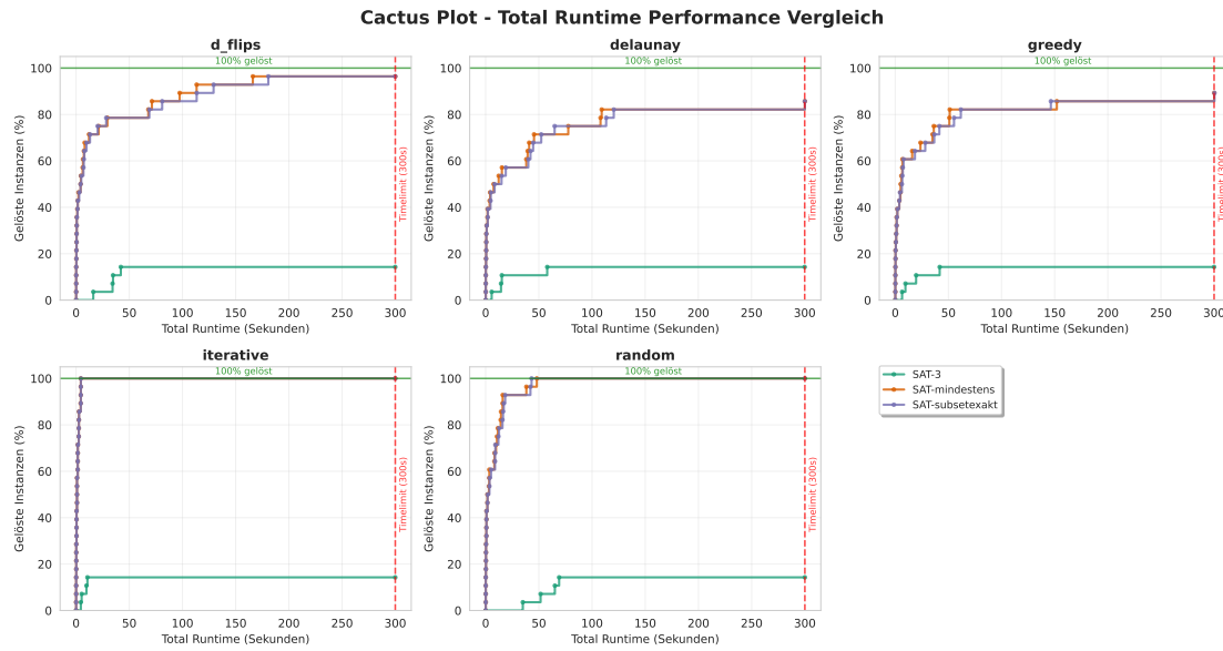
Abbildung 4.10: die besten Ergebnisse der verschiedenen Gradbeschränkungen in einem SAT Solver.
