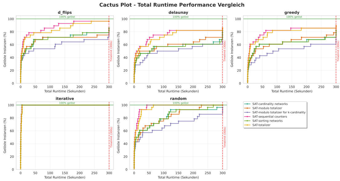
Abbildung 4.8: Die exact Methode für die Gradbeschränkung in einem SAT Solver, wurde mit verschiedenen Kardinalitätsbedingung getestet.
