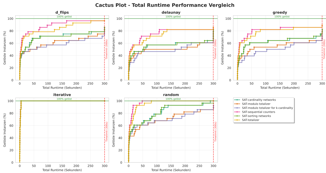
Abbildung 4.9: Die atleast Methode für die Gradbeschränkung in einem SAT Solver, wurde mit verschiedenen Kardinalitätsbedingung getestet.
