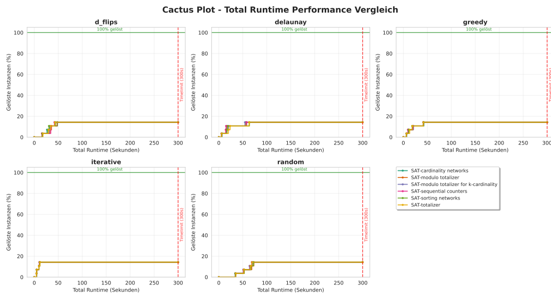
Abbildung 4.7: Die subset Methode für die Gradbeschränkung in einem SAT Solver, wurde mit verschiedenen Kardinalitätsbedingung getestet.
