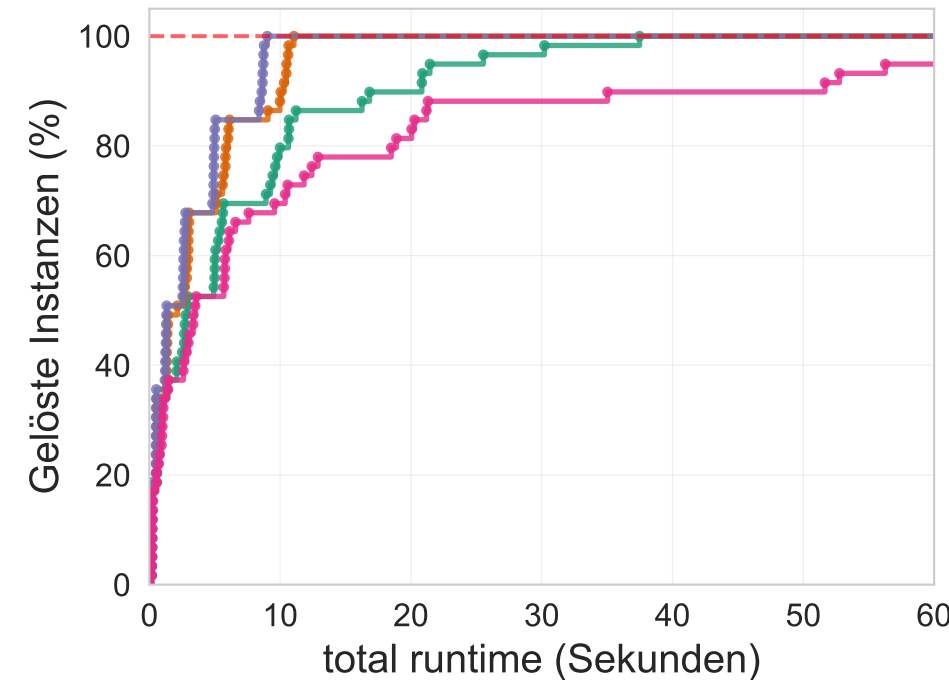
Gesamt
