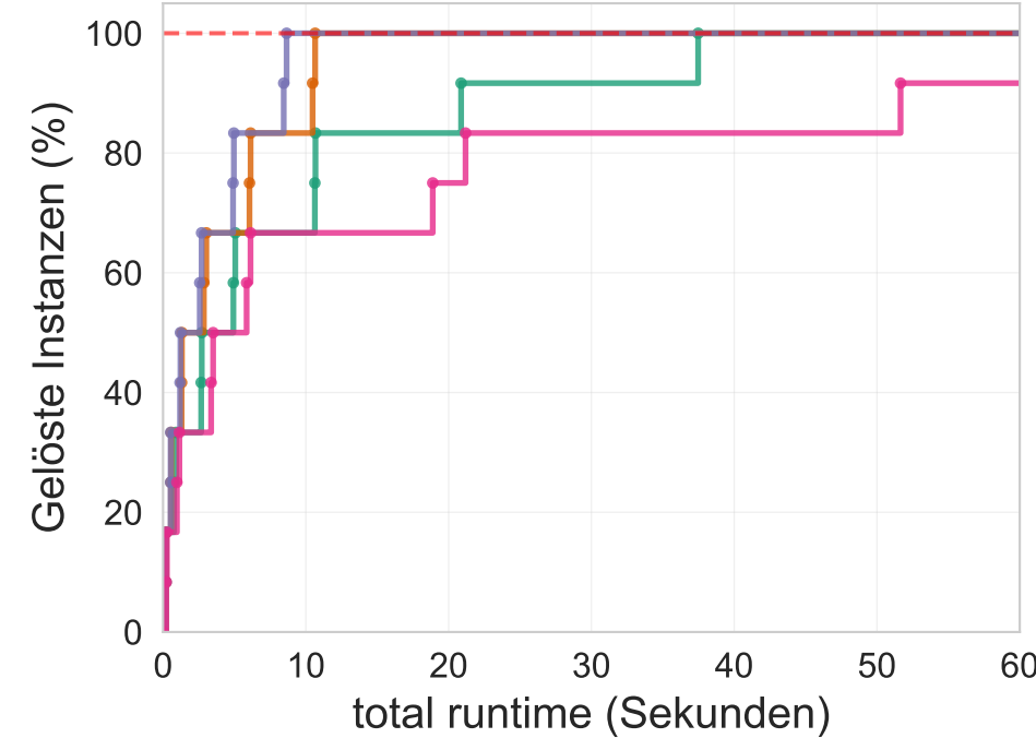
Gesamt
