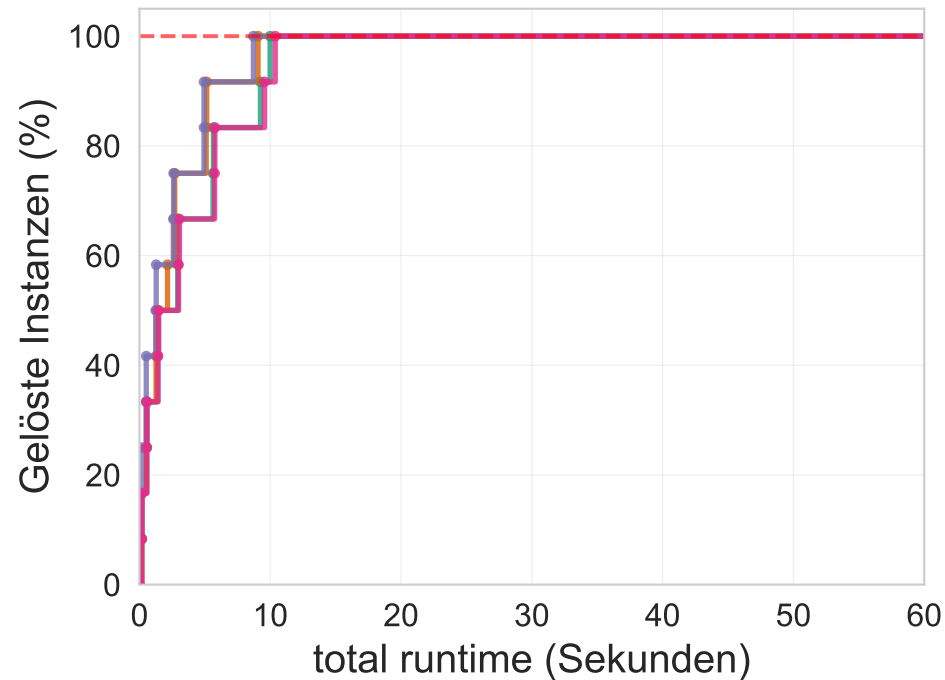
Iterativ
