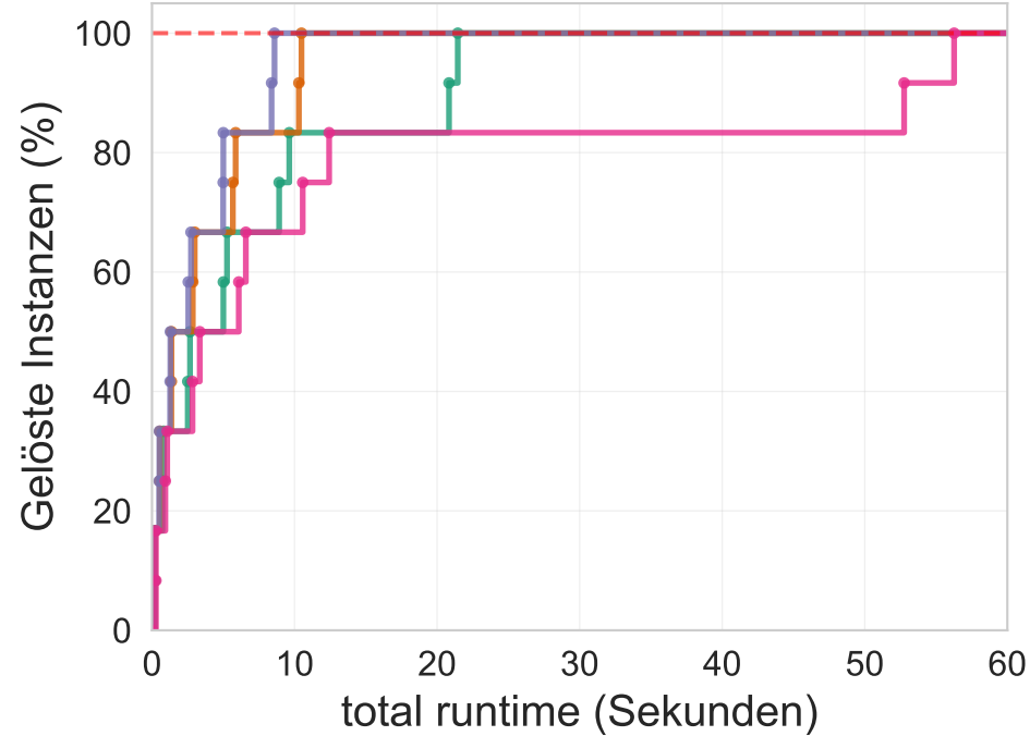
Iterativ
