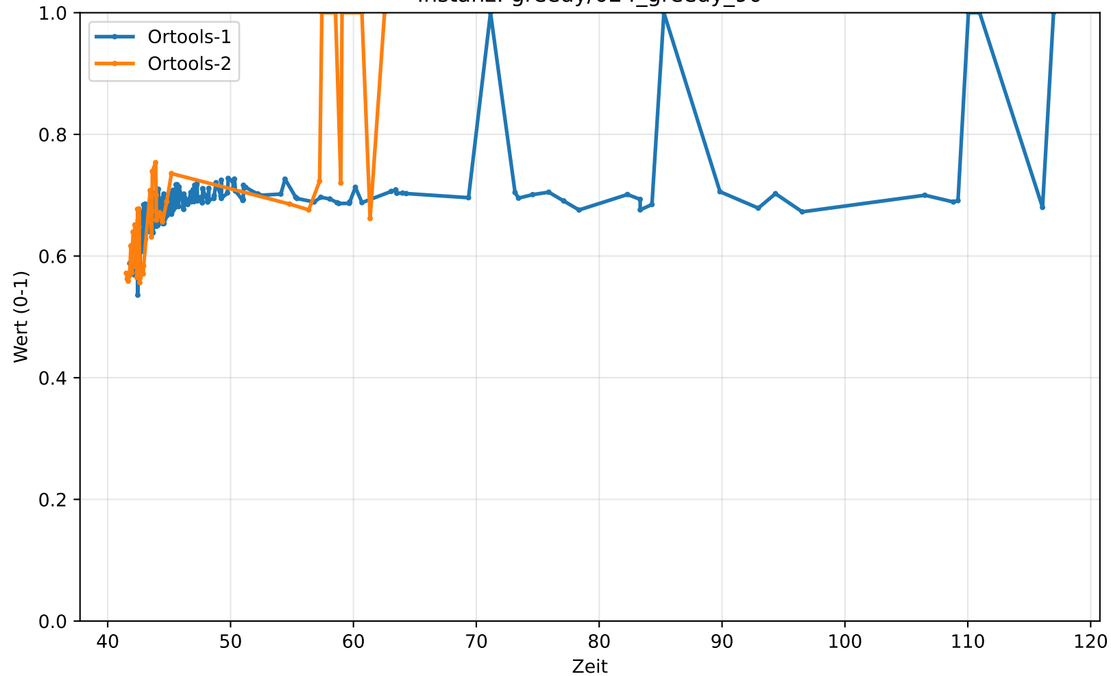
Instanz: greedy/024_greedy_90
