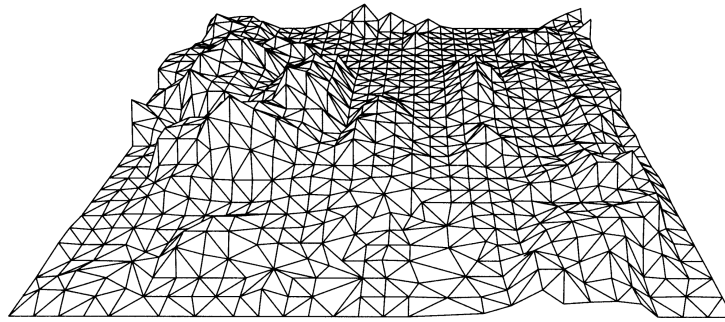
Abbildung 1.2.: Ein Beispiel für Höhendaten durch eine Triangulation aus [8, p. 183]
