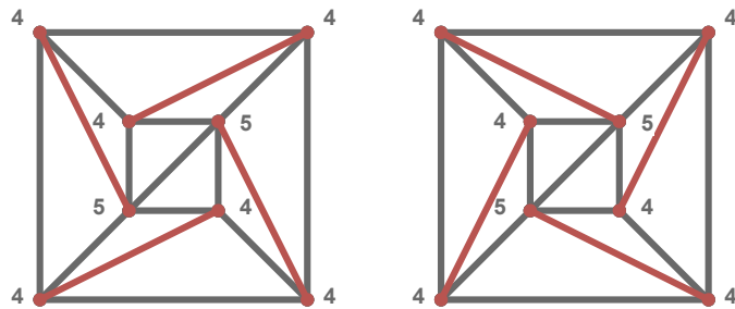
Abbildung 3.6.: Eine Ja-Instanz mit zwei möglichen Lösungen. Die Zahlen an den Knoten geben hierbei den Sollgrad an. Die roten kanten sind jene die in den Lösungen unterschiedlich sind.
