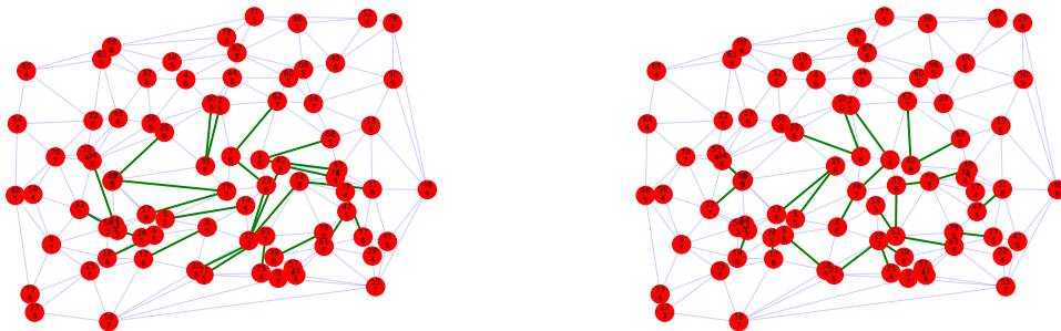
Abbildung 4.4.: Eval8 Anzahl Lösungen Delaunay
