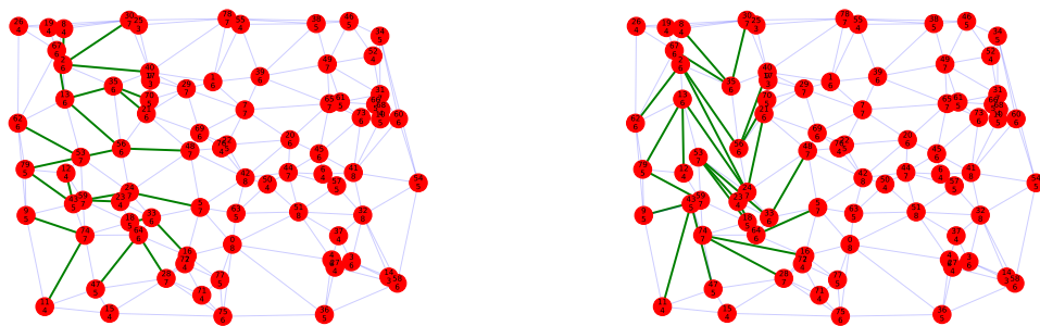
Abbildung 4.5.: Eval8 Anzahl Lösungen Greedy
