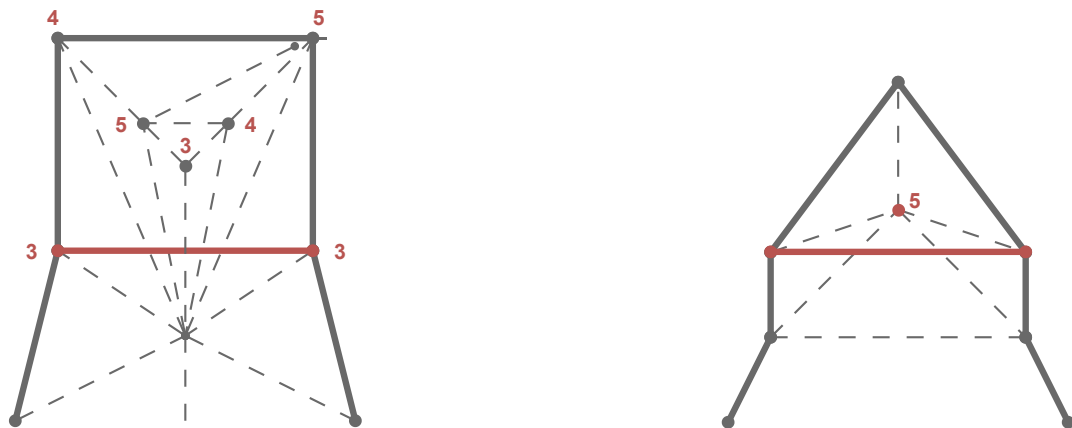
Abbildung 3.2.: Zwei Teilinstanzen, in welcher die rote Kante ausgeschlossen werden kann. Links da die Gradsumme die Anzahl der Kanten unterschreitet und rechts da der mittlere rote Knoten nicht genügend Kanten erzeugen könnte.
