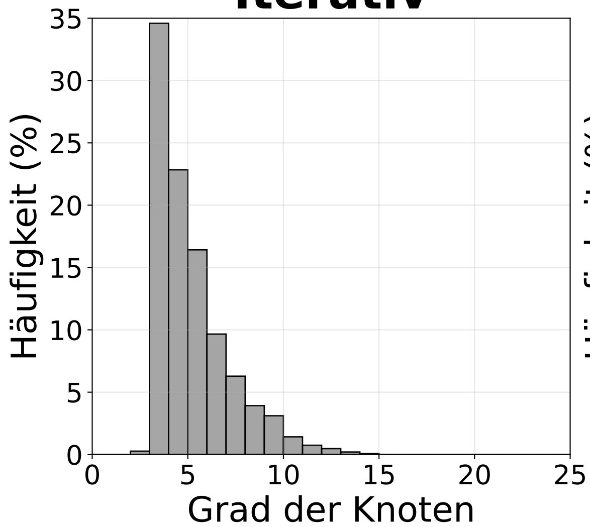
Iterativ
