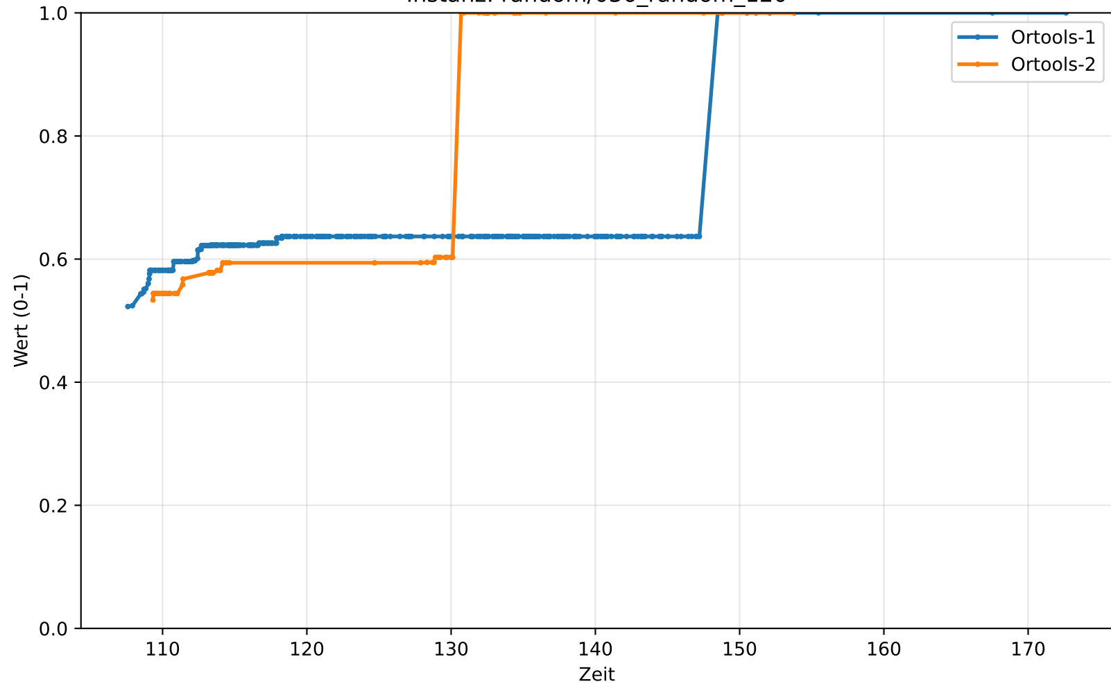
Instanz: random/036_random_120
