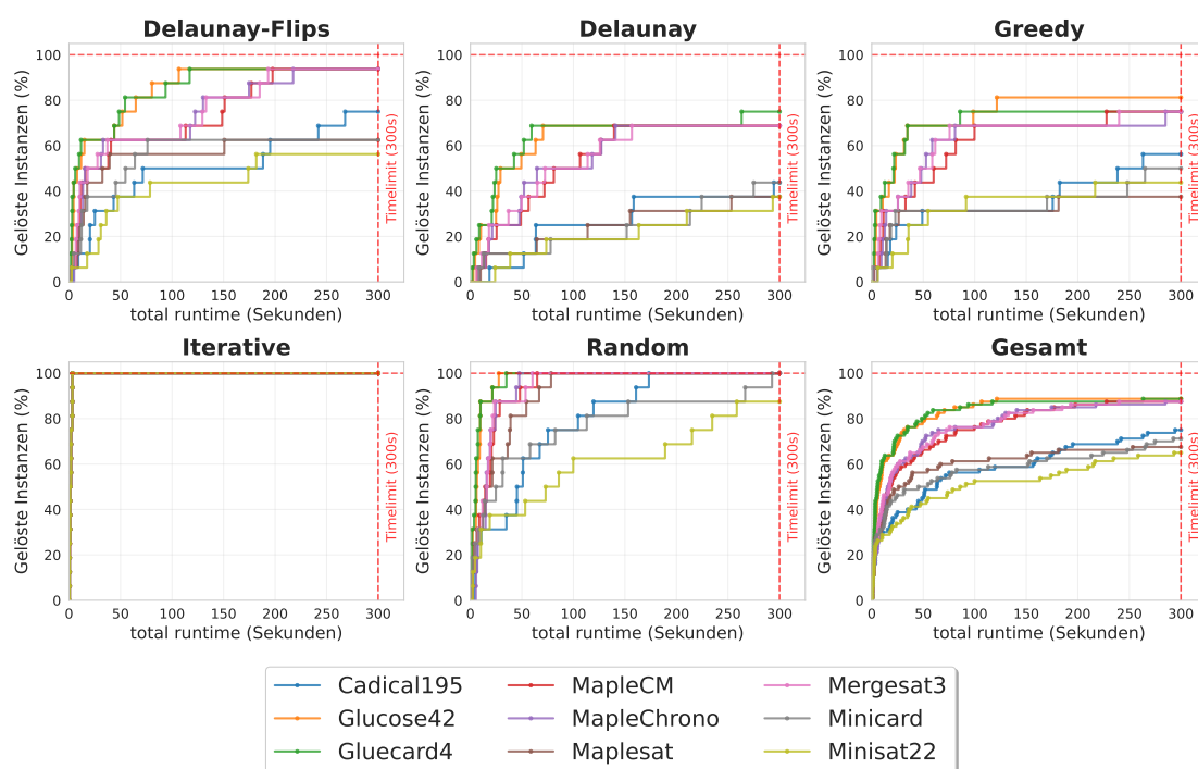
Abbildung 6.2.: In dieser Abbildung sind die Laufzeiten der verschiedenen SAT-Solver für die verschiedenen Instanzen zu sehen. Hierbei ist klar erkennbar das Gluecard4 und Glucose42 die besten Ergebnisse erzielen.
