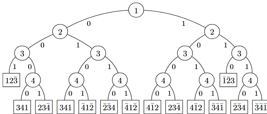
Abbildung 5.1.: Ein Baum welcher die Möglichen Entscheidungen eines SAT-Solvers darstellt. Jeder Ast entspricht Belegungen der Literale
