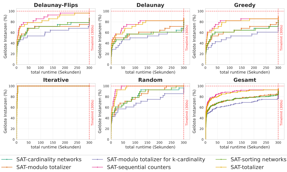
Abbildung C.1.: Gelöste Instanzen und Laufzeit unter verschiedenen Ansätzen, die Kardinalitätsbedingungen ( \sum_{vw \in E} x_{vw} = \deg^*(v) in CNF zu kodieren; höher/weiter links ist besser. Man sieht, dass sequential counters am besten funktionieren, gefolgt von totalizer .
