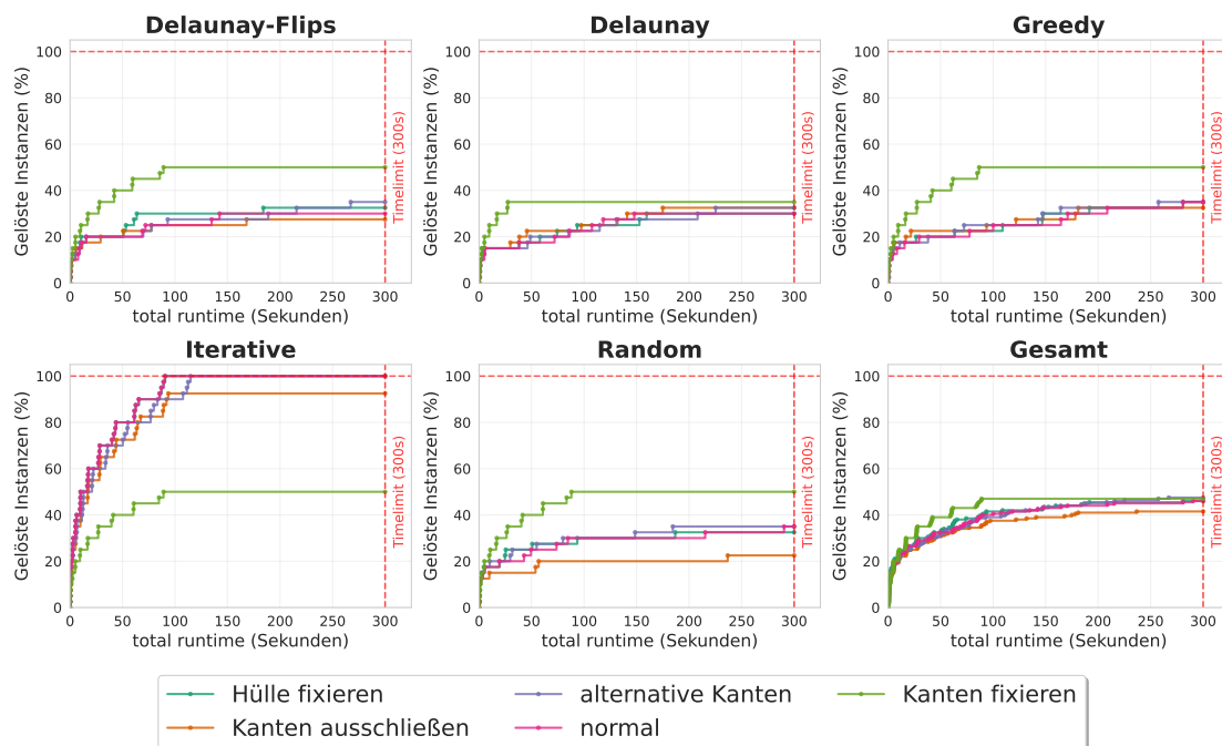
Abbildung D.4.: Eval1 Gurobi
