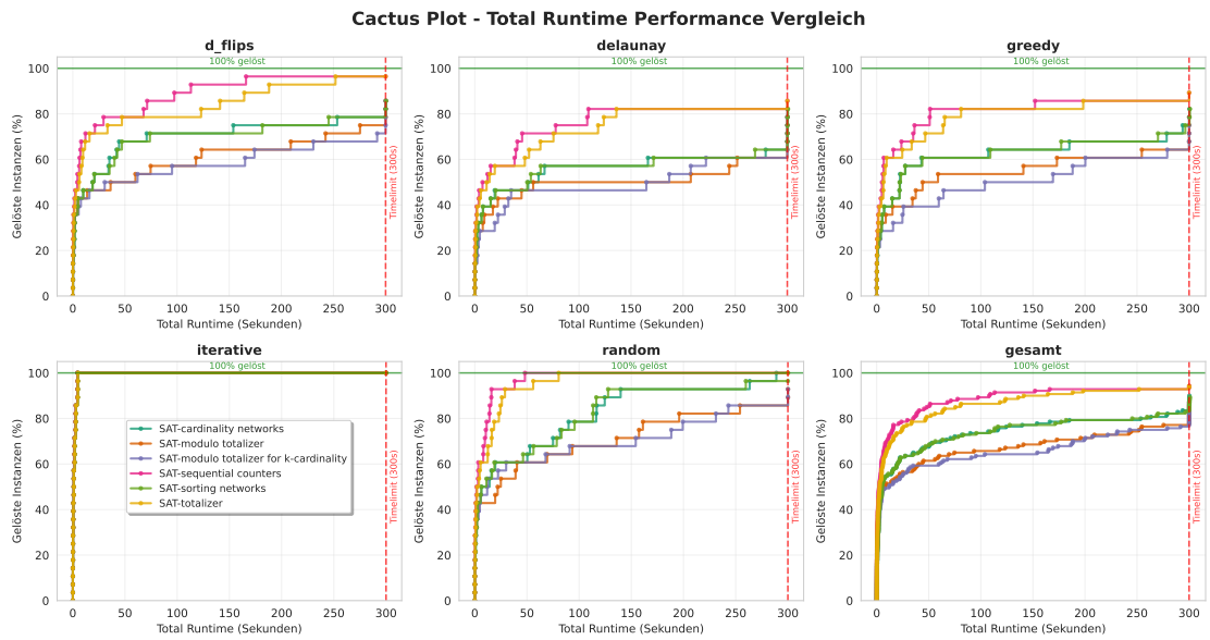
Abbildung A.2.: Die atleast Methode für die Gradbeschränkung in einem SAT Solver, wurde mit verschiedenen Kardinalitätsbedingung getestet.
