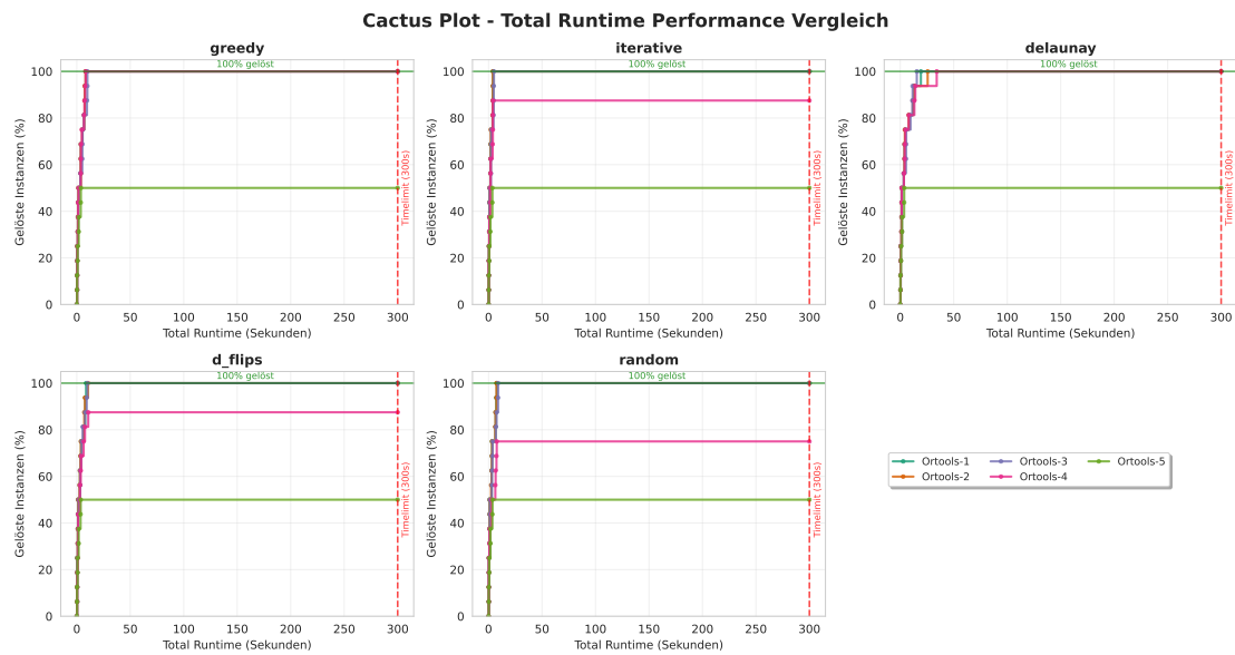
Abbildung B.3.: Eval1 OrTools
