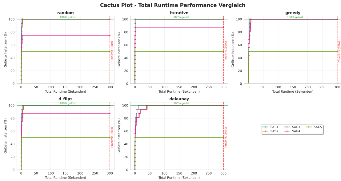
Abbildung B.2.: Eval1 Sat
