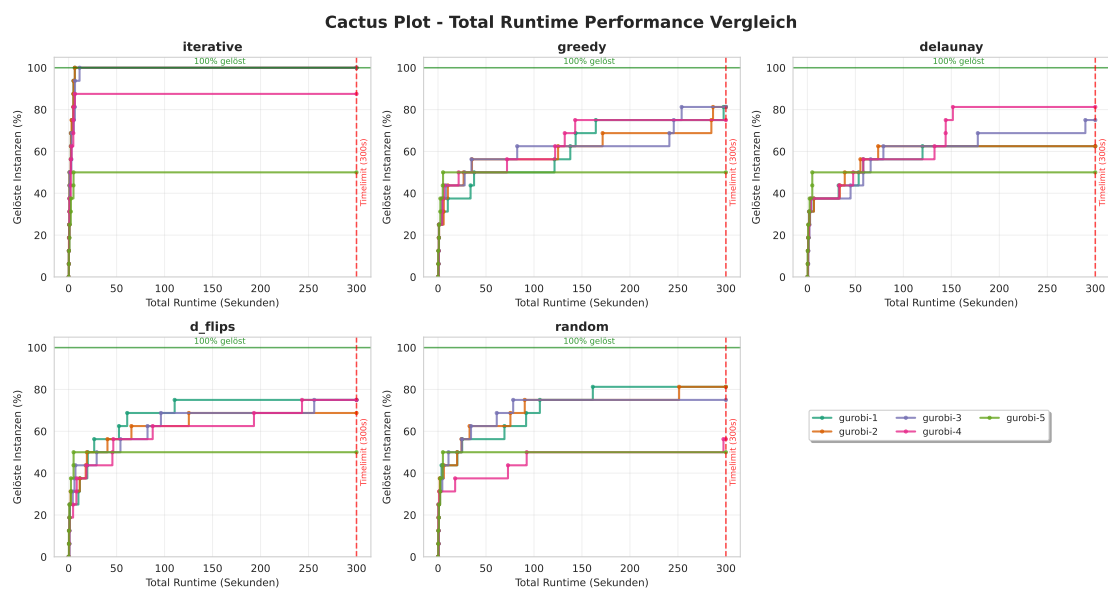
Abbildung B.4.: Eval1 Gurobi
