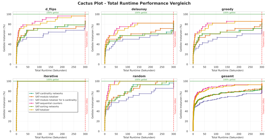
Abbildung A.1.: Die exact Methode für die Gradbeschränkung in einem SAT Solver, wurde mit verschiedenen Kardinalitätsbedingung getestet.
