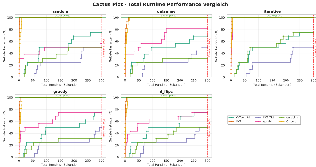
Abbildung 4.2.: Eval1 Gesamt
