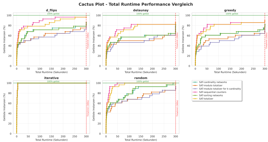
Abbildung 4.3: Die atleast Methode für die Gradbeschränkung in einem SAT Solver, wurde mit verschiedenen Kardinalitätsbedingung getestet.
