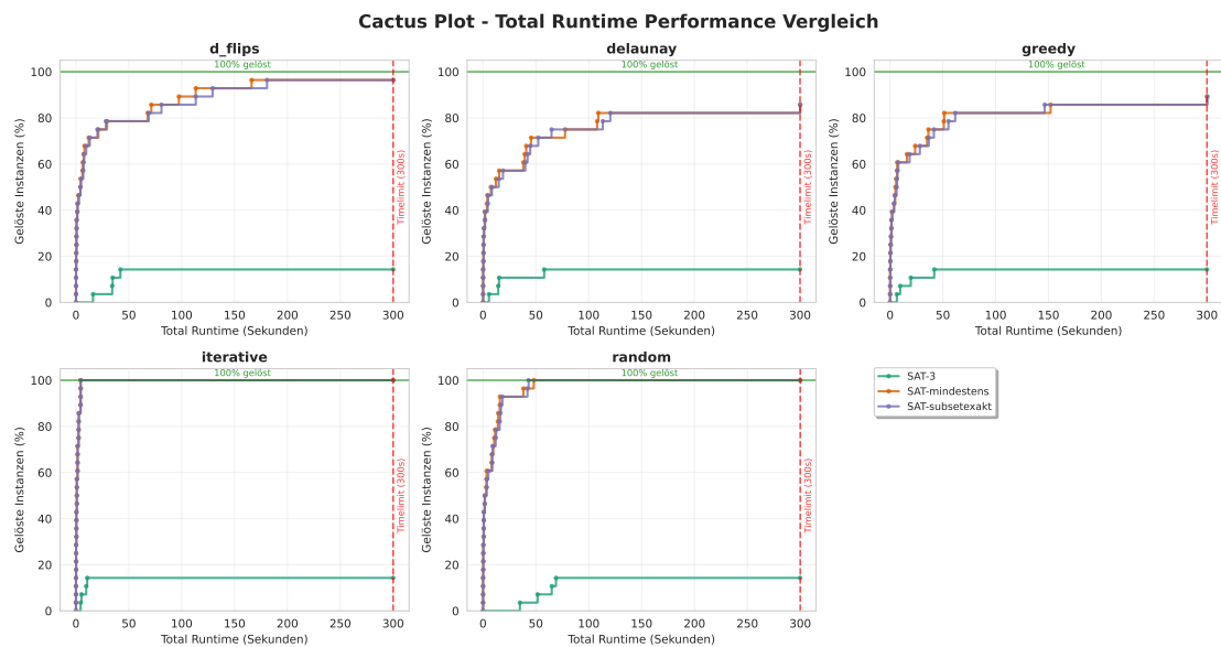
Abbildung 4.4: die besten Ergebnisse der verschiedenen Gradbeschränkungen in einem SAT Solver.
