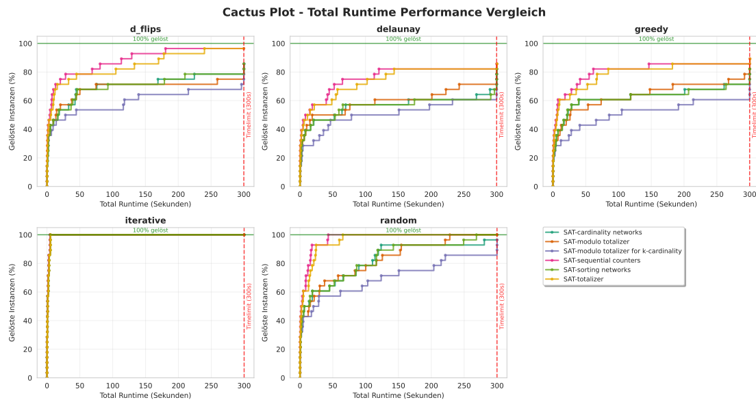
Abbildung 4.2: Die exact Methode für die Gradbeschränkung in einem SAT Solver, wurde mit verschiedenen Kardinalitätsbedingung getestet.
