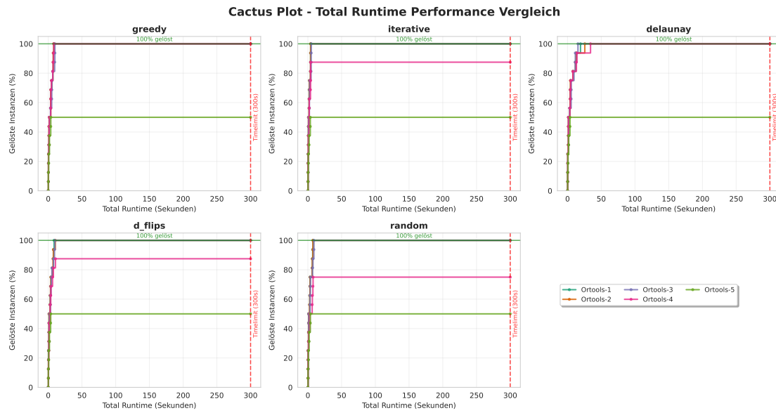
Abbildung 4.4.: Eval1 OrTools
