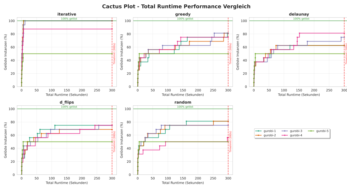
Abbildung 4.5.: Eval1 Gurobi
