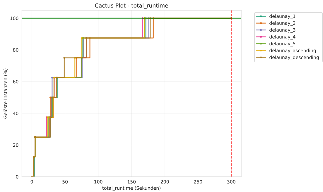
Abbildung 4.6: Eval2 Permutation Instanz
