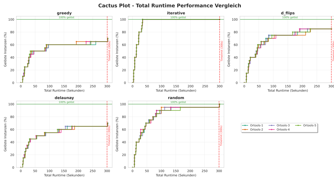
Abbildung 4.8: Eval7 Selbe Solver Selbe Instanz OrTools
