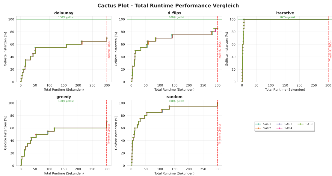
Abbildung 4.9: Eval7 Selbe Solver Selbe Instanz SAT
