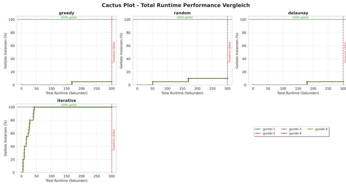
Abbildung 4.7: Eval7 Selbe Solver Selbe Instanz Gurobi
