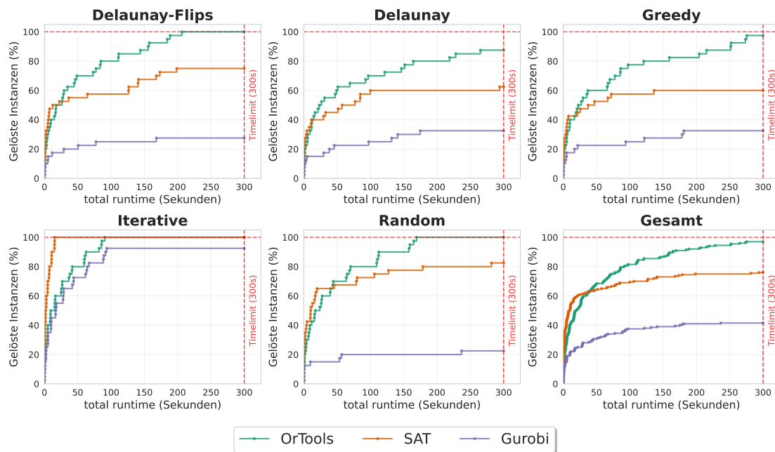
Abbildung 6.3.: In dieser Abbildung werden für die sechs verschiedenen Ansätze die besten Solver verglichen. Hierbei ist klar erkennbar das OrTools die besten Ergebnisse erzielt
