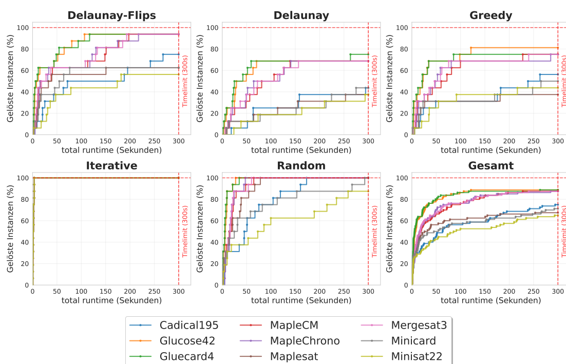
Abbildung 6.2.: In dieser Abbildung sind die Laufzeiten der verschiedenen SAT-Solver für die verschiedenen Instanzen zu sehen. Hierbei ist klar erkennbar dass Gluecard4 und Glucose42 die besten Ergebnisse erzielen.
