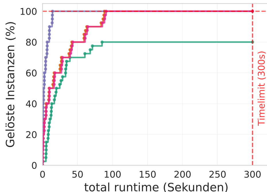
Iterativ
