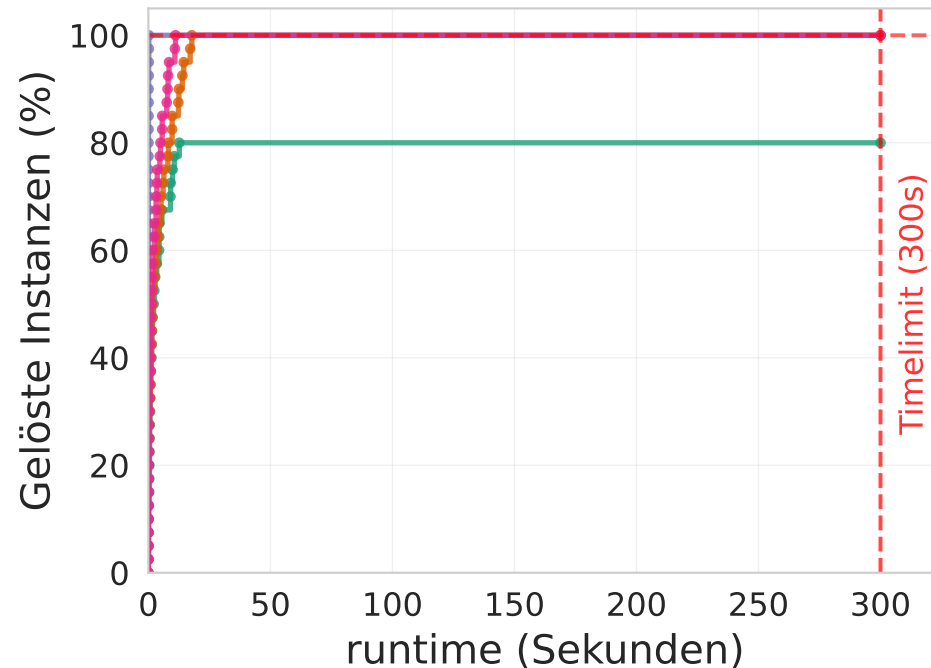
Iterativ
