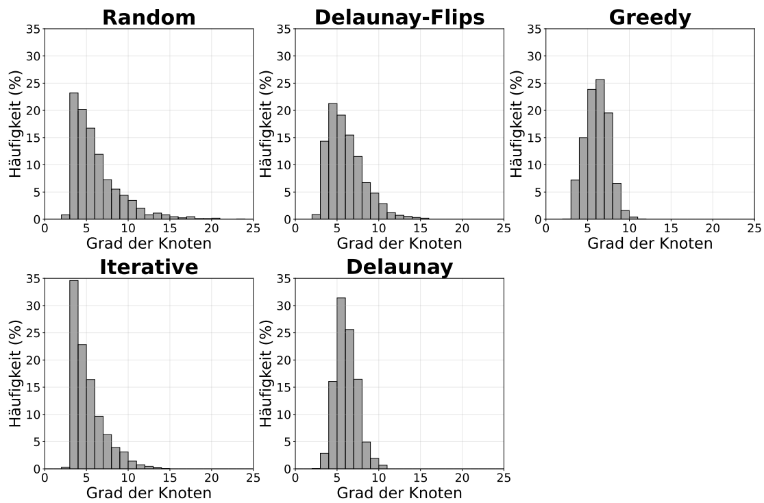
Abbildung 5.10.: In dieser Abbildung ist die Gradverteilung der Knoten pro Instanz zu sehen.
