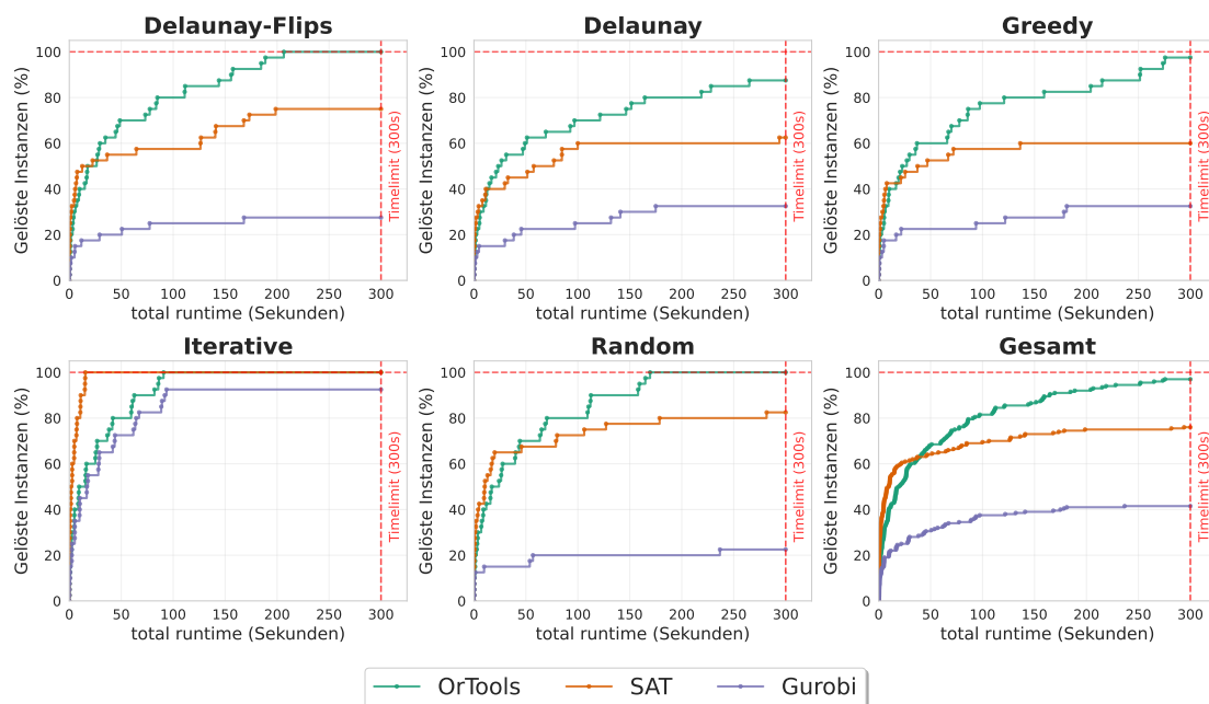
Abbildung 5.3.: In dieser Abbildung werden für die sechs verschiedenen Ansätze die besten Solver verglichen. Hierbei ist klar erkennbar das OrTools die besten Ergebnisse erzielt
