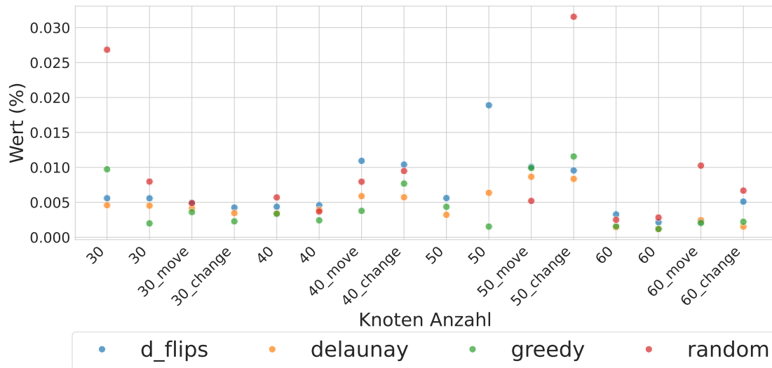
Abbildung 5.8.: In der Abbildung sind die Relativen Anzahlen der Erfolgreichen Propagation zu sehen. Das bedeutet die Anzahl der Erfolgreichen Propagation geteilt durch die Anzahl der Propagation Aufrufe.
