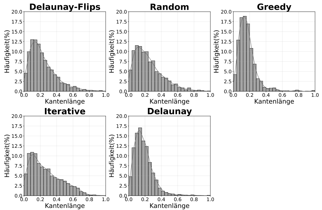
Abbildung 5.11.: In dieser Abbildung ist die Verteilung der Kantenlängen pro Instanz zu sehen. Dabei sind die Kantenlängen normiert, sodass sie zwischen 0 und 1 liegen. Dafür wurde alle Kantenlängen durch die maximale Kantenlänge geteilt.
