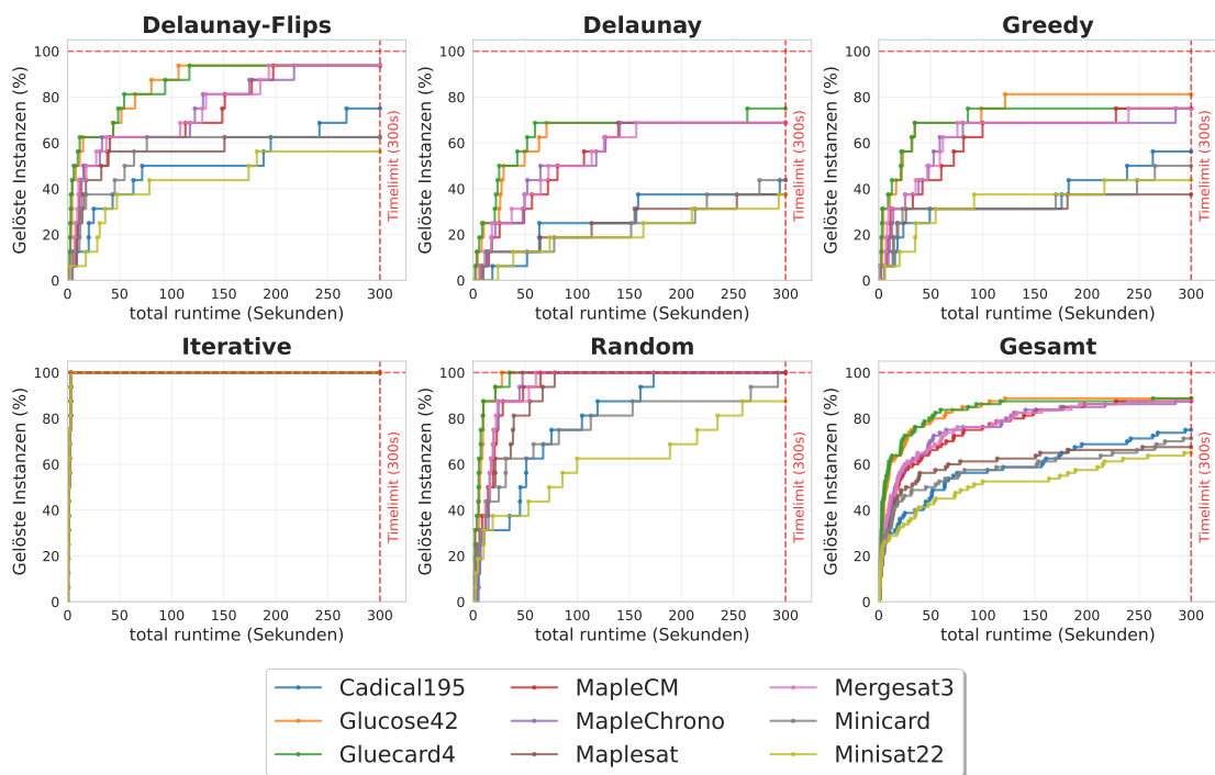
Abbildung 5.2.: In dieser Abbildung sind die Laufzeiten der verschiedenen SAT-Solver für die verschiedenen Instanzen zu sehen. Hierbei ist klar erkennbar dass Gluecard4 und Glucose42 die besten Ergebnisse erzielen.
