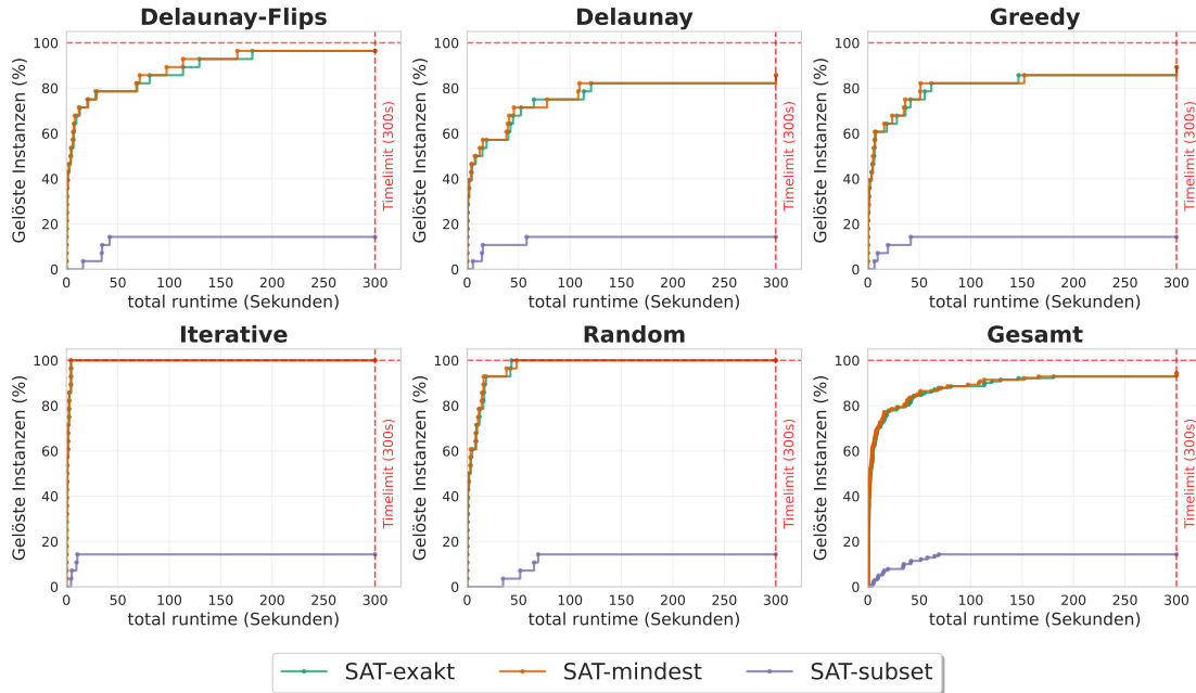
Abbildung 5.1.: In der Abbildung werden für alle Instanzen Arten die drei Kardinalitätsbeschränkungen verglichen. Die subset Methode ist die schlechteste, da sie nur für kleine Instanzen funktioniert. Die anderen beiden Methoden unterscheiden sich nicht signifikant.
