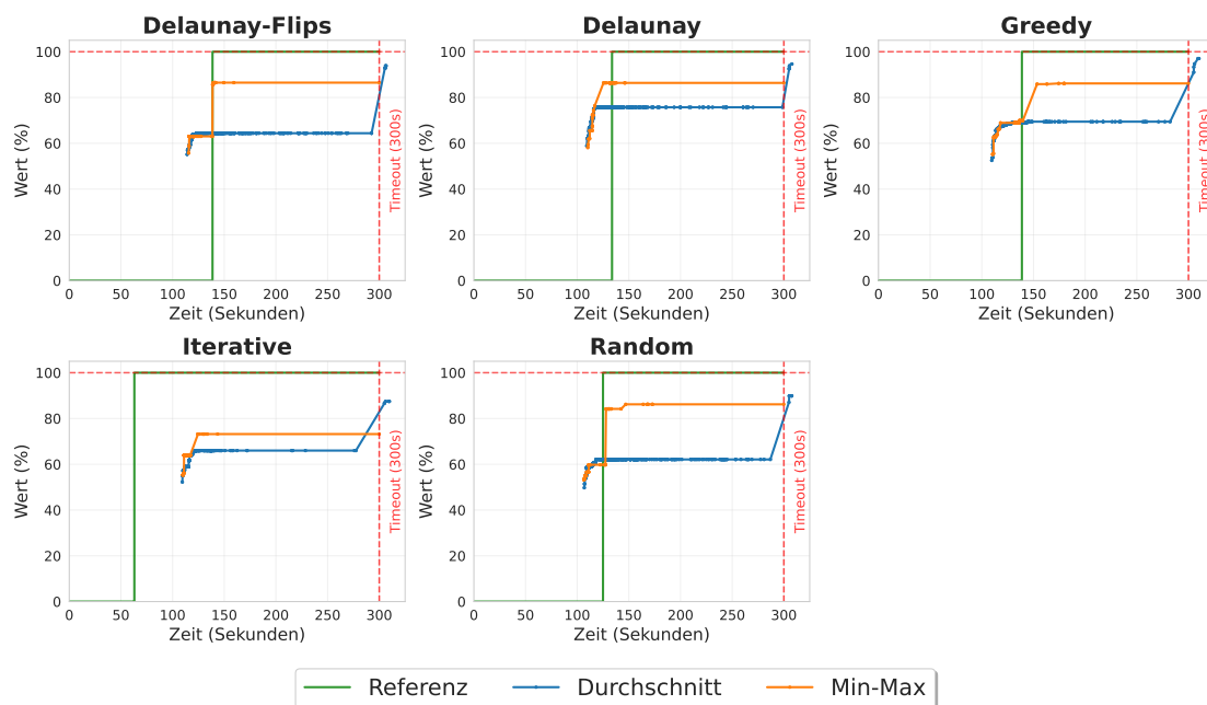
Abbildung 5.6.: Eine Nein-Instanz mit 120 Knoten. Hier werden zwei verschiedene Ansätze mit Zielfunktionen mit einem Referenzsolver aus Abschnitt 5.6 verglichen. Der Durchschnittsansatz ist in den meisten Fällen besser als der Min-Max Ansatz. Es ist nicht erkennbar ob der Zielfunktionen Ansatz besser oder schlechter als der Referenzsolver ist.
