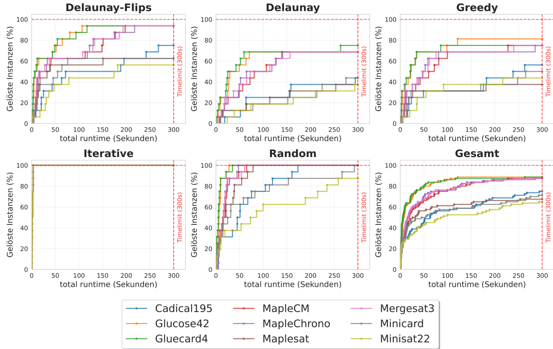
Abbildung 4.2.: Eval3 Gesamt
