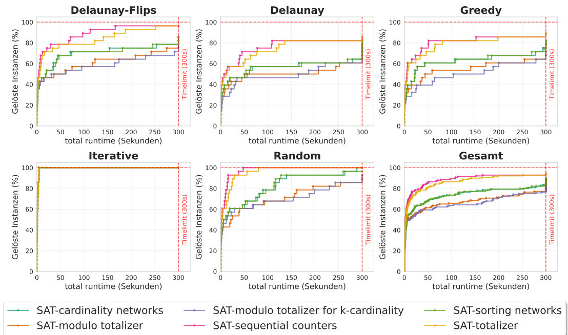
Abbildung C.2.: Die atleast Methode für die Gradbeschränkung in einem SAT Solver, wurde mit verschiedenen Kardinalitätsbedingung getestet.
