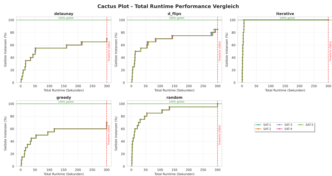
Abbildung B.3.: Es ist zu sehen das SAT bei der gleichen Instanz und den gleichen Beschränkungen bei Mehrmaligen durchlaufen die gleichen Laufzeiten hat.
