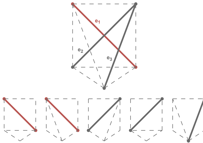
Abbildung 3.4.: Ein Vollständiger Graph mit allen möglichen Triangulierung. Die Kanten e_2 und e_3 sind Schnittekanten von e_1 . Es ist zu sehen das e_1 oder eine der Schnittekanten aktiv sein muss damit eine Triangulierung möglich ist.
