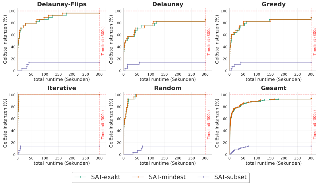
Abbildung 4.1.: die besten Ergebnisse der verschiedenen Gradbeschränkungen in einem SAT Solver.
