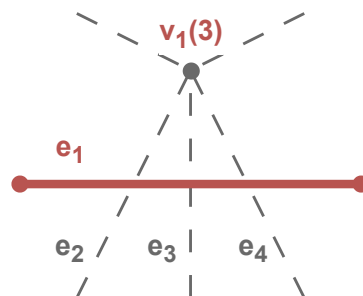
Abbildung 3.4: In der Abbildung hat der Knoten v_1 einen Sollgrad von 3. Da die Kante e_1 drei von fünf möglichen Kanten blockiert, kann v_1 seinen Sollgrad nicht erreichen. Daher kann e_1 ausgeschlossen werden.
