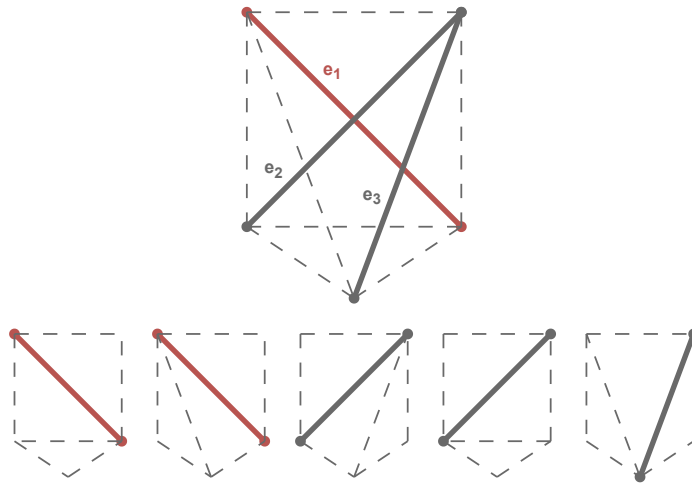
Abbildung 3.1: Ein Vollständiger Graph mit allen möglichen Triangulation. Die Kanten e_2 und e_3 sind Schnittkanten von e_1 . Es ist zu sehen das e_1 oder eine der Schnittkanten aktiv sein muss damit eine Triangulation möglich ist.
