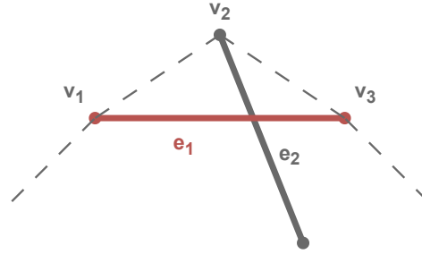
Abbildung 3.2: Abhängig von dem Sollgrad von v_2 kann entschieden werden ob e_1 aktiv oder nicht aktiv sein muss. Sollte \deg^*(v_2) = 2 sein, dann muss e_1 aktiv sein damit alle Kanten wie e_2 nicht aktiv sein können. Sollte \deg^*(v_2) > 2 sein, dann muss e_1 nicht aktiv sein damit der Sollgrad erreicht werden kann.
