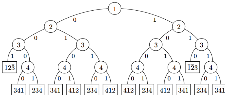
Abbildung 3.6: Ein Baum, welcher die möglichen Entscheidungen eines SAT-Solvers darstellt. Jeder Ast entspricht einer Belegung der Literale
