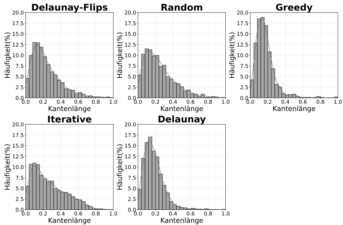
Abbildung 6.11.: In dieser Abbildung ist die Verteilung der Kantenlängen pro Instanz zu sehen. Dabei sind die Kantenlängen normiert, sodass sie zwischen 0 und 1 liegen. Dafür wurde alle Kantenlängen durch die maximale Kantenlänge geteilt.
