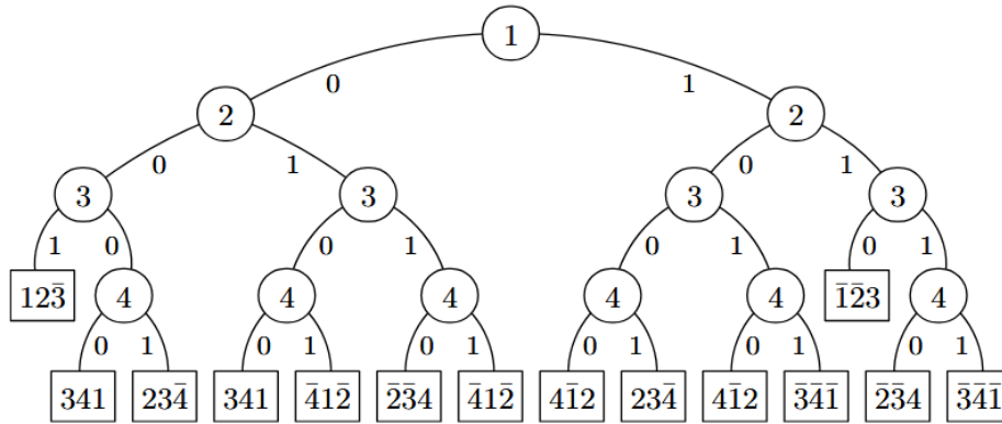
Abbildung 3.5.: Ein Baum welcher die Möglichen Entscheidungen eines SAT-Solvers darstellt. Jeder Ast entspricht einer Belegung der Literale
