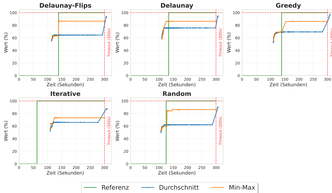
Abbildung 6.6.: Eine Nein-Instanz mit 120 Knoten. Hier werden zwei verschiedene Ansätze mit Zielfunktionen mit einem Referenzsolver aus Abschnitt 6.6 verglichen. Der Durchschnittsansatz ist in den meisten Fällen besser als der Min-Max Ansatz. Es ist nicht erkennbar ob der Zielfunktionen Ansatz besser oder schlechter als der Referenzsolver ist.
