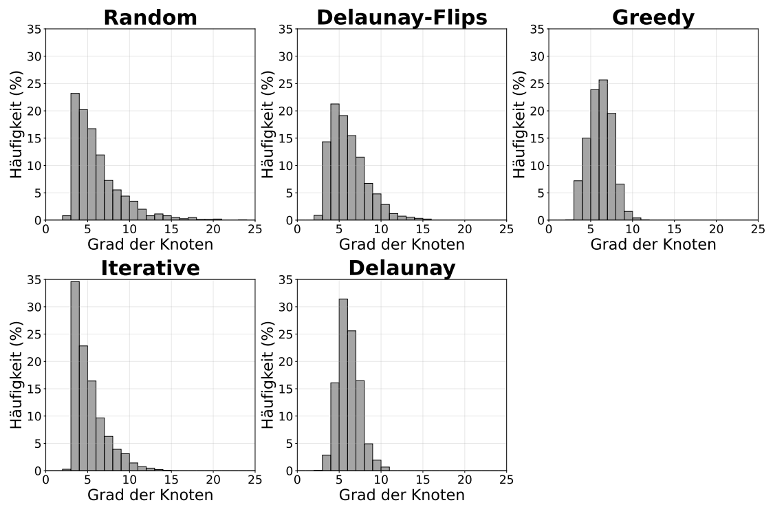
Abbildung 6.10.: In dieser Abbildung ist die Gradverteilung der Knoten pro Instanz zu sehen.
