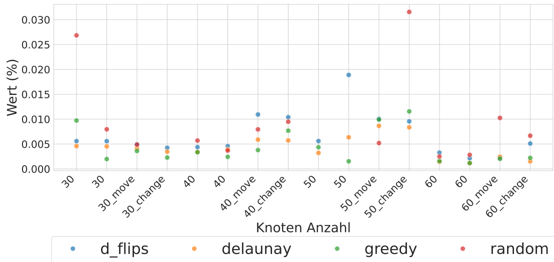
Abbildung 6.8.: In der Abbildung sind die Relativen Anzahlen der Erfolgreichen Propagation zu sehen. Das bedeutet die Anzahl der Erfolgreichen Propagation geteilt durch die Anzahl der Propagation Aufrufe.
