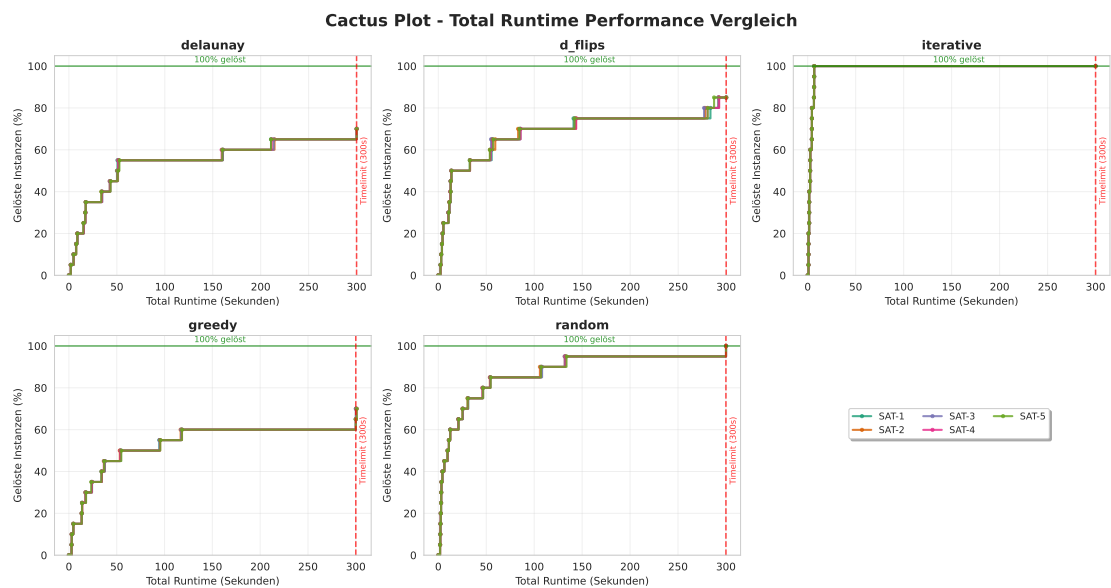
Abbildung 4.4: Eval7 Selbe Solver Selbe Instanz SAT
