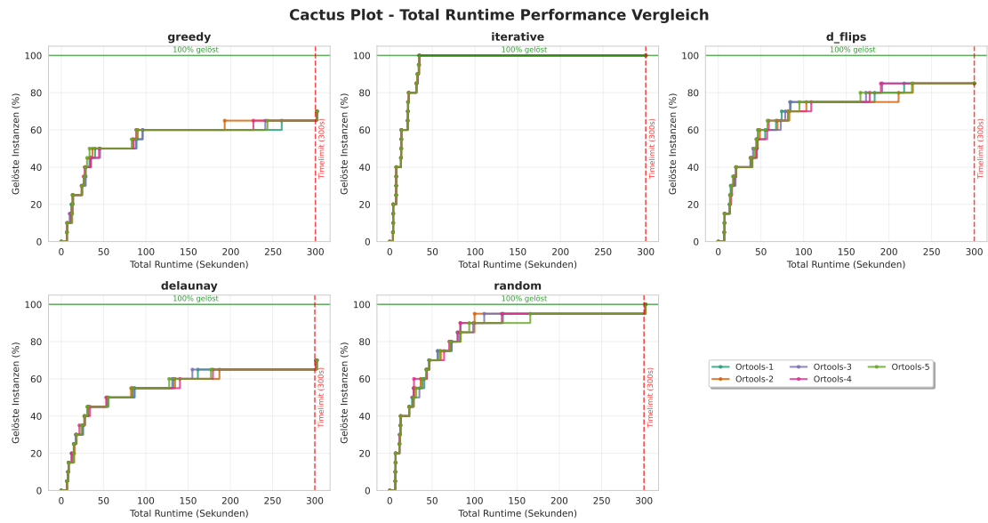
Abbildung 4.3: Eval7 Selbe Solver Selbe Instanz OrTools
