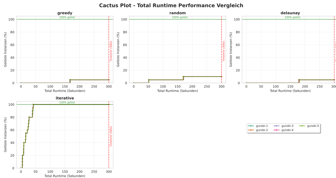
Abbildung 4.2: Eval7 Selbe Solver Selbe Instanz Gurobi
