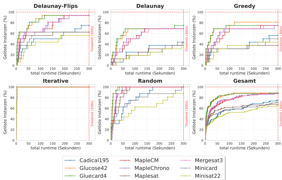
Abbildung 6.2.: In dieser Abbildung sind die Laufzeiten der verschiedenen SAT-Solver für die verschiedenen Instanzen zu sehen. Hierbei ist klar erkennbar, dass Gluecard4 und Glucose42 die besten Ergebnisse erzielen.
