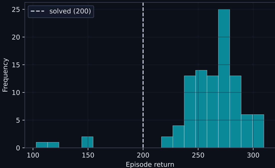
PPO best seed 4 — 262 \pm 34
